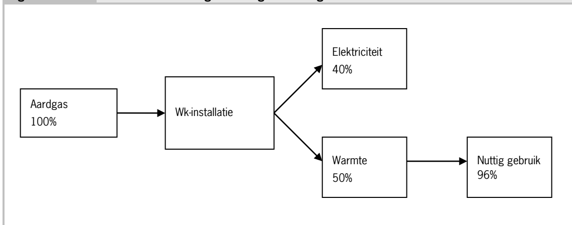
Figuur B1.1 Schematische weergave energiebenutting uit wk-installaties tuinders
