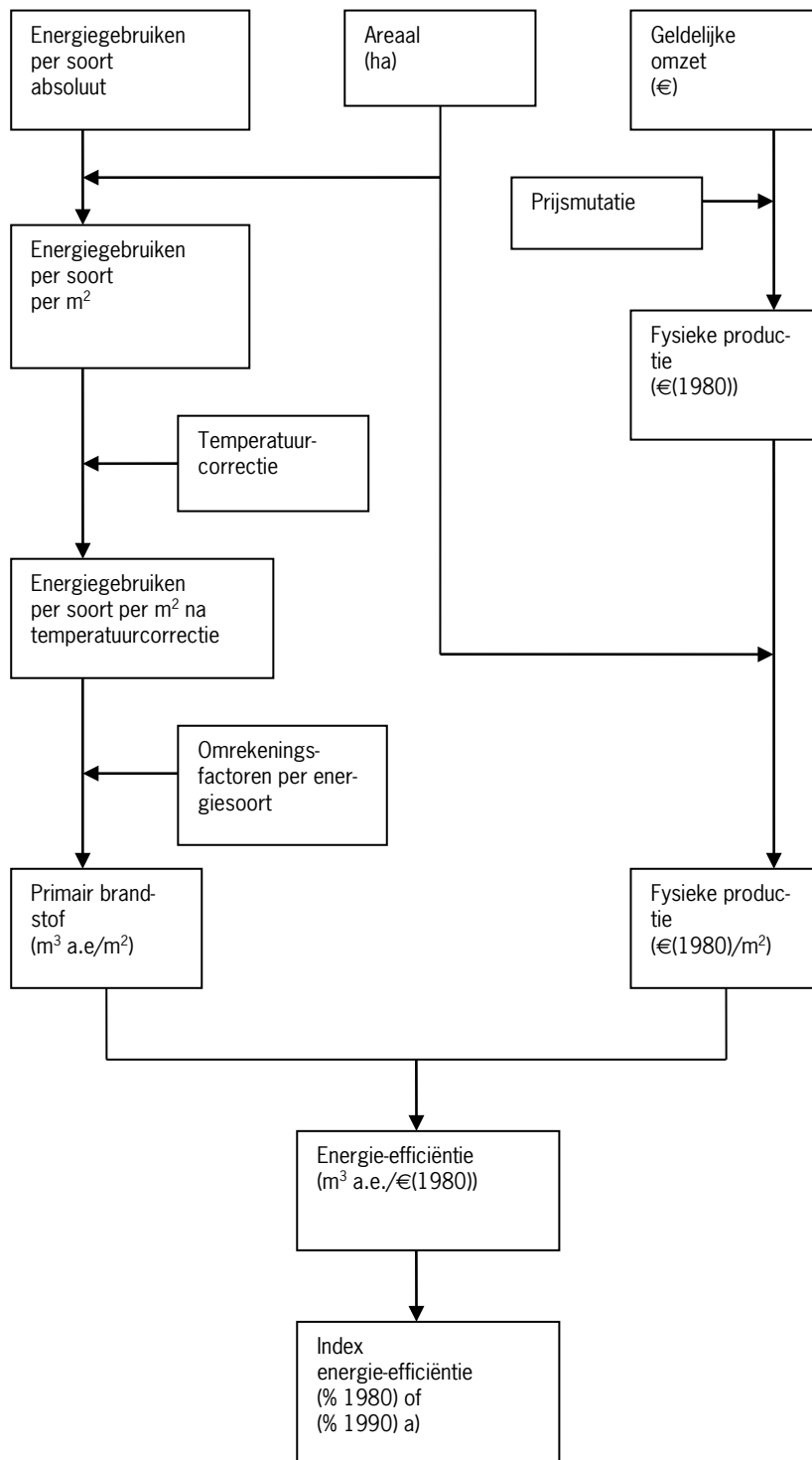
Figuur 2.1 Schematische weergave bepaling energie-efficiëntie productieglastuinbouw
