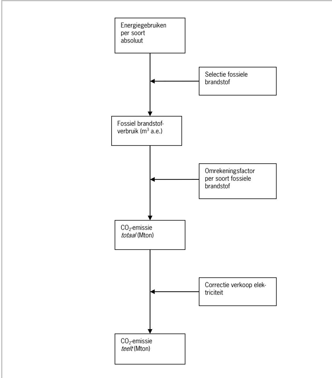
Figuur 2.2 Schematische weergave bepaling CO 2 -emissie glastuinbouw
