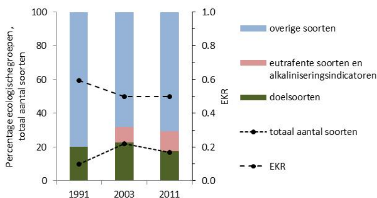
Figuur 5.7.4 Verloop van de procentuele hoeveelheid van indicatorgroepen, totaal aantal soorten en EKR voor de vegetatie in het Elpermeer.
