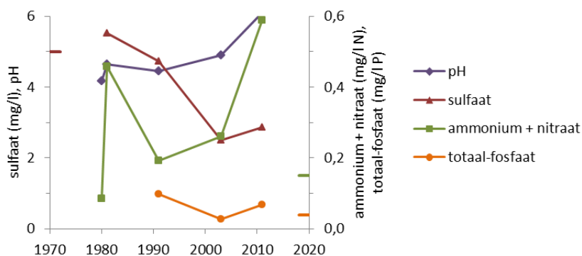
Figuur 5.14.2 Veranderingen van jaargemiddelden van geselecteerde chemische variabelen in het Langeveen. De streepjes langs de assen zijn rapportagegrenzen. Vanaf 1991 zijn er meestal 4 waarnemingen per jaar, daarvoor minder.
