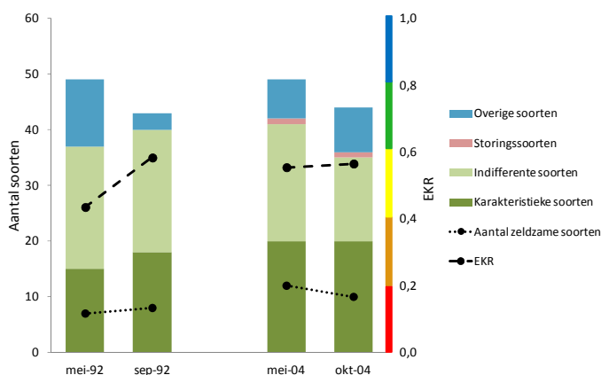
Figuur 5.9.7 Verloop van het aantal soorten macrofauna, met onderscheid naar categorieën volgens Duursema (1996), zeldzame soorten (Nijboer & Verdonschot 2001) en de EKR in de Gouden Ploeg. Op de gekleurde balk langs de rechter verticale as kan de bijbehorende kwaliteitsklasse volgens Tabel 2.12 worden afgelezen.
