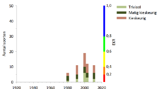
Figuur 5.11.6 Verloop van het aantal soorten sieralgen in het ven Kampsheide, met onderscheid naar kieskeurigheid. Op het gekleurde balkje langs de rechter verticale as kan de bijbehorende kwaliteitsklasse volgens Tabel 2.15 worden afgelezen.
