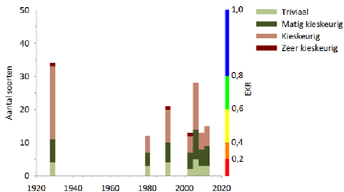
Figuur 5.19.7 Verloop van het aantal soorten sialgen in het Zandveen, met onderscheid naar kieskeurigheid. Op het gekleurde balkje langs de rechter verticale as kan de bijbehorende kwaliteitsklasse volgens Tabel 2.15 worden afgelezen.
