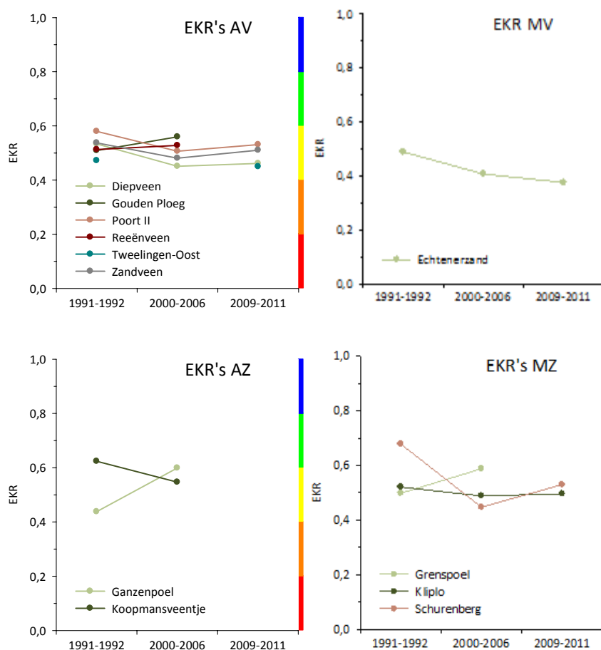
Figuur 3.25 Gemiddelde EKR van macrofauna voor ieder ven per type in drie perioden. De gekleurde balk rechts geeft de vijf kwaliteitsklassen volgens Tabel 2.12 aan: rood is slecht, oranje is ontoereikend, geel is matig, groen is goed en blauw is zeer goed.
