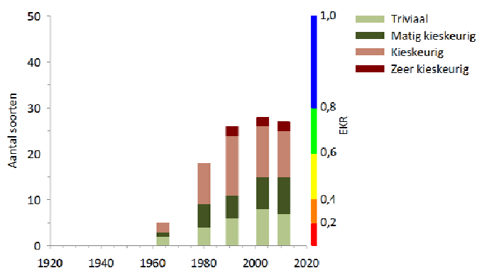
Figuur 5.9.6 Verloop van het aantal soorten sieralgen in de Gouden Ploeg, met onderscheid naar kieskeurigheid. Op het gekleurde balkje langs de rechter verticale as kan de bijbehorende kwaliteitsklasse volgens Tabel 2.15 worden afgelezen.
