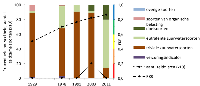
Figuur 5.16.5 Verloop van de procentuele hoeveelheid van ecologische groepen, EKR en aantal zeldzame soorten (x10) in de tellingen van kiezelwieren in netplanktonmonsters uit het Reeënveen. Het gekleurde balkje langs de rechter verticale as geeft de vijf kwaliteitsklassen volgens Tabel 2.12 aan.
