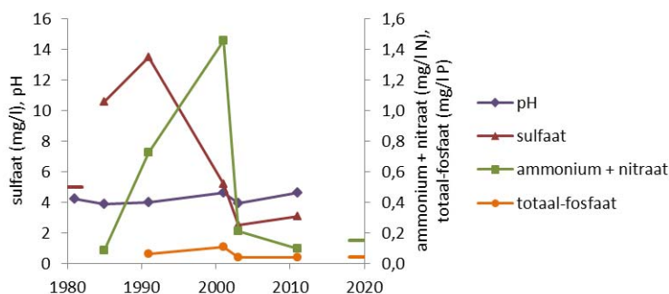
Figuur 5.13.2 Veranderingen van jaargemiddelden van geselecteerde chemische variabelen in het Koopmansveentje. De streepjes langs de assen zijn rapportagegrenzen. Vanaf 1991 zijn er meestal 4 waarnemingen per jaar, daarvoor minder.
