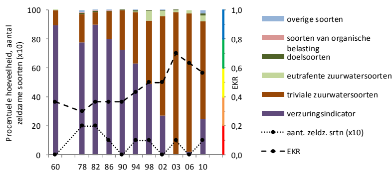
Figuur 5.6.5 Verloop van de procentuele hoeveelheid van ecologische groepen, EKR en aantal zeldzame soorten (x10) in de tellingen van kiezelwieren uit netplanktonmonsters uit het ven in het Echtenerzand. Het gekleurde balkje langs de rechter verticale as geeft de vijf kwaliteitsklassen volgens Tabel 2.12 aan.
