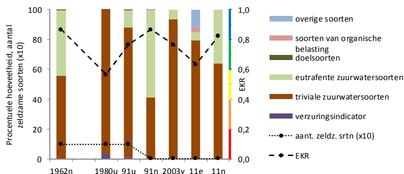
Figuur 5.18.5 Verloop van de procentuele hoeveelheid van ecologische groepen, EKR en aantal zeldzame soorten (x10) in de tellingen van kiezelwieren in De Tweelingen-Oost. e = epifyten (aangroeiisel), n = netplankton, u = uitknijpsel, v = netplankton + uitknijpsel. Het gekleurde balkje langs de rechter verticale as geeft de vijf kwaliteitsklassen volgens Tabel 2.12 aan.
