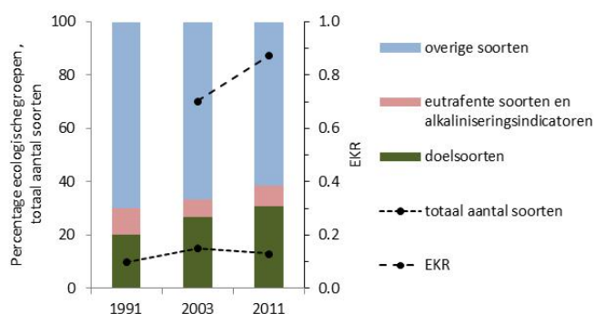
Figuur 5.18.4 Verloop van de procentuele hoeveelheid van indicatorgroepen, totaal aantal soorten en EKR op basis van de macrofyten soortensamenstelling voor de vegetatie in De Tweelingen
