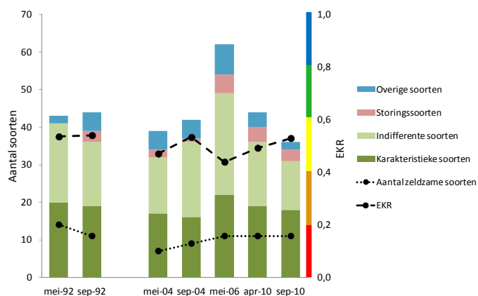
Figuur 5.19.8 Verloop van het aantal soorten macrofauna, met onderscheid naar categorieën volgens Duursema (1996), zeldzame soorten (Nijboer & Verdonshot 2001) en de EKR in het Zandveen. Op de gekleurde balk langs de rechter verticale as kan de bijbehorende kwaliteitsklasse volgens Tabel 2.12 worden afgelezen.
