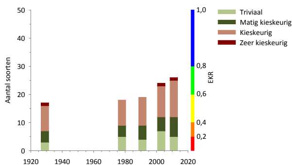
Figuur 5.16.6 Verloop van het aantal soorten sieralgen in het Reeënnen, met onderscheid naar kieskeurigheid. Op het gekleurde balkje langs de rechter verticale as kan de bijbehorende kwaliteitsklasse volgens Tabel 2.15 worden afgelezen.
