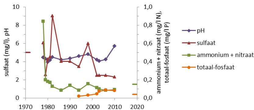
Figuur 5.15.4 Veranderingen van jaargemiddelden van geselecteerde chemische variabelen in de grootste poel van Poort 2. De streepjes langs de assen zijn rapportagegrenzen. Vanaf 1991 zijn er meestal 4 waarnemingen per jaar, daarvoor minder.
