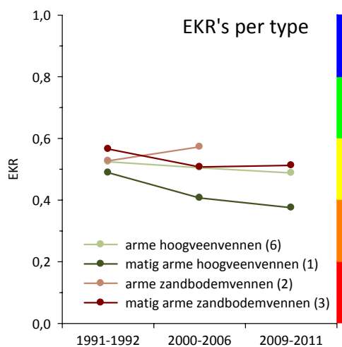
Figuur 3.24 Gemiddelde EKR van macrofauna per type in drie perioden. De gekleurde balk rechts geeft de vijf kwaliteitsklassen volgens Tabel 2.12 aan: rood is slecht, oranje is ontoereikend, geel is matig, groen is goed en blauw is zeer goed. Tussen haakjes het aantal vennen.
