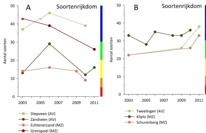
Figuur 3.21 Ontwikkeling van de soortenrijkdom van sieralgen in tussentijds bemonsterde vennen in de periode 2003-2011. A. Drie van de vier vennen vertonen in 2006 een piek in de soortenrijkdom. De Grenspoel laat een consistente afname zijn in diversiteit. B. De soortenrijkdom stijgt in alle drie licht tot sterk. In het ven Tweelingen neemt het aantal soorten in twee jaar tijd met bijna 50% toe. Het gekleurde balkje rechts geeft de bijbehorende vijf kwaliteitsklassen van de KRW aan: rood is slecht, oranje is ontoereikend, geel is matig, groen is goed en blauw is zeer goed.
