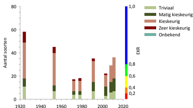
Figuur 5.17.6 Verloop van het aantal soorten sieralgen in Schurenberg, met onderscheid naar kieskeurigheid. Op het gekleurde balkje langs de rechter verticale as kan de bijbehorende kwaliteitsklasse volgens Tabel 2.15 worden afgelezen.
