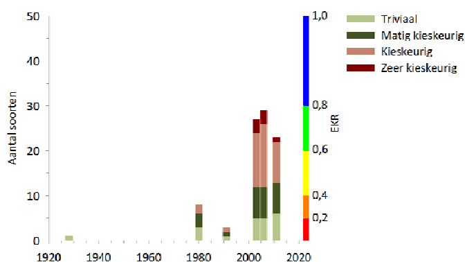
Figuur 5.14.6 Verloop van het aantal soorten sieralgen in het Langeveen, met onderscheid naar kieskeurigheid. Op het gekleurde balkje langs de rechter verticale as kan de bijbehorende kwaliteitsklasse volgens Tabel 2.15 worden afgelezen.
