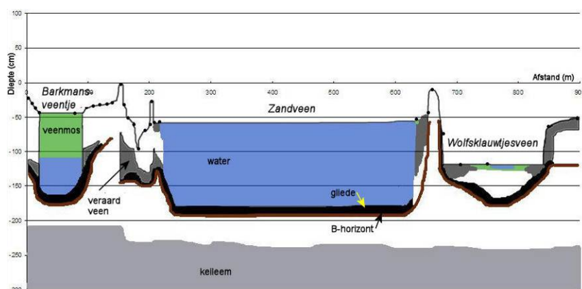
Figuur 5.19.2. Doorsnede door Barkmansveentje, Zandveen en Wolfsklauwtjesveen (Lanting 2009, Baaijens e.a. 2011).
