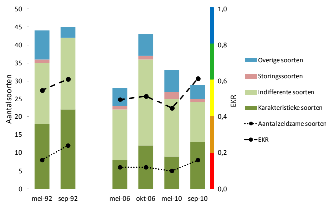
Figuur 5.15.9 Verloop van het aantal soorten macrofauna, met onderscheid naar categorieën volgens Duursema (1996), zeldzame soorten (Nijboer & Verdonschot 2001) en de EKR in Poort 2. Op de gekleurde balk langs de rechter verticale as kan de bijbehorende kwaliteitsklasse volgens Tabel 2.12 worden afgelezen.
