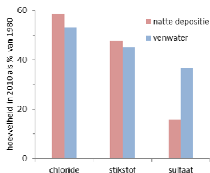
Figuur 3.9 Veranderingen van de relatieve hoeveelheden van chloride, (ammonium- en nitraat-)stikstof en sulfaat in de natte depositie te Witteveen/Valthermond (volgens Tabel 3.1) en de gemiddelde concentraties in 18 Drentse vennen (Tabel 3.12).
