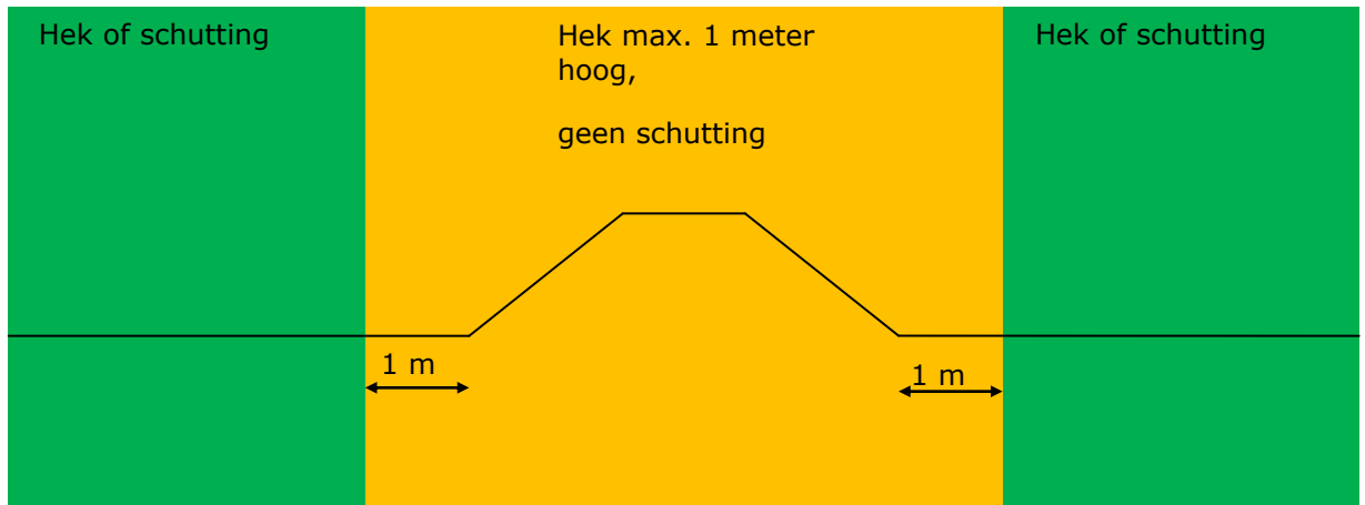
Figuur 5 niet direct waterkerende kering
