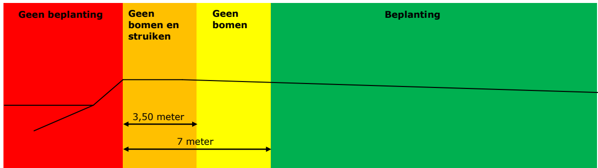
Figuur 2: verheelde en aangeheelde regionale waterkering
