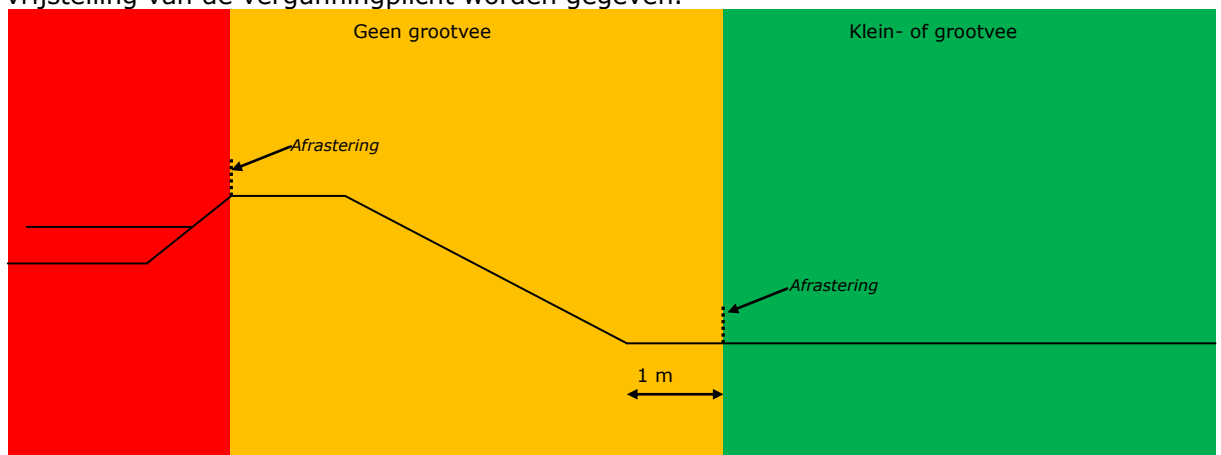
Figuur 6 niet verheelde of aangeheelde waterkering
