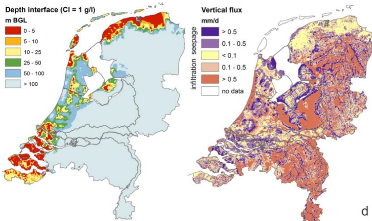
Figuur 3. De diepte van het brak-zout grensvlak, CI-concentratie = 1000 mg/l. (links) en de kwel (blauw) en infiltratieflux (rood) (rechts, modelresultaat NHI 3.0 (De Lange e.a., 2014)).
