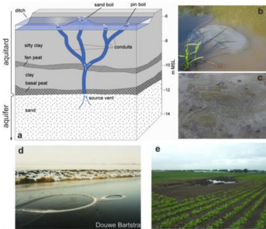
Figuur 2. (boven) Drie verschillende typen zoute kwel die verschillen in flux en zoutgehalte, (links) schematische voorstelling van een wel in de deklaag en enkele foto's van wellen; (b) zandwel, (c) methaangas dat via wellen ontsnapt, (d) wellen en ijs, (e) een wel op het land (De Louw, 2013).
