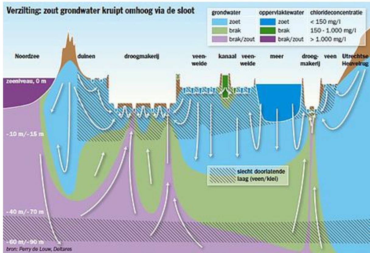
Figuur 4. Vereenvoudigd van regionaal west-oost profiel met grondwaterstromingspatronen en zoutgehaltes van grondwater, ter hoogte van de Haarlemmermeerpolder. Verzilting van het grondwatersysteem vindt op regionale schaal plaats omdat het gemiddeld polderpeil enkele meters lager ligt dan het gemiddeld zeeniveau. In de droogmakerij vindt opkegeling van zout grondwater plaats door de wellen die in de polder aanwezig zijn. De zoute wellen zijn hier dominant in de verzilting van het oppervlaktewater.
