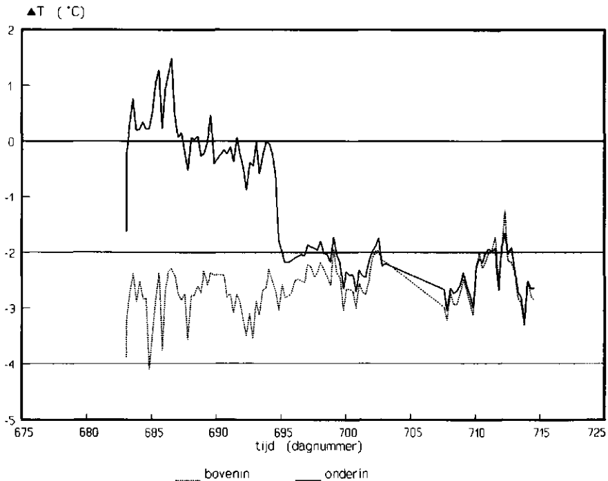
Figuur 8 Het temperatuursverschil tussen drukkamer en respectievelijk bovenin en onderin het filtermateriaal in het midden van het biofilter in de periode oktober tot november 1992. Figure 8 Difference in temperature between filter material (top and bottom) and pressure cabin from October till November 1992.
