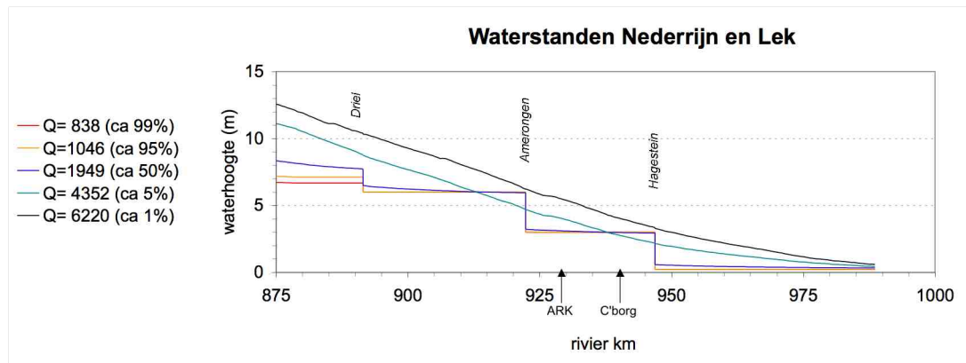
Figuur 2.3: Waterstandsverloop Nederrijn-Lek bij verschillende afvoeren (berekeningen op basis van SOBEK).
