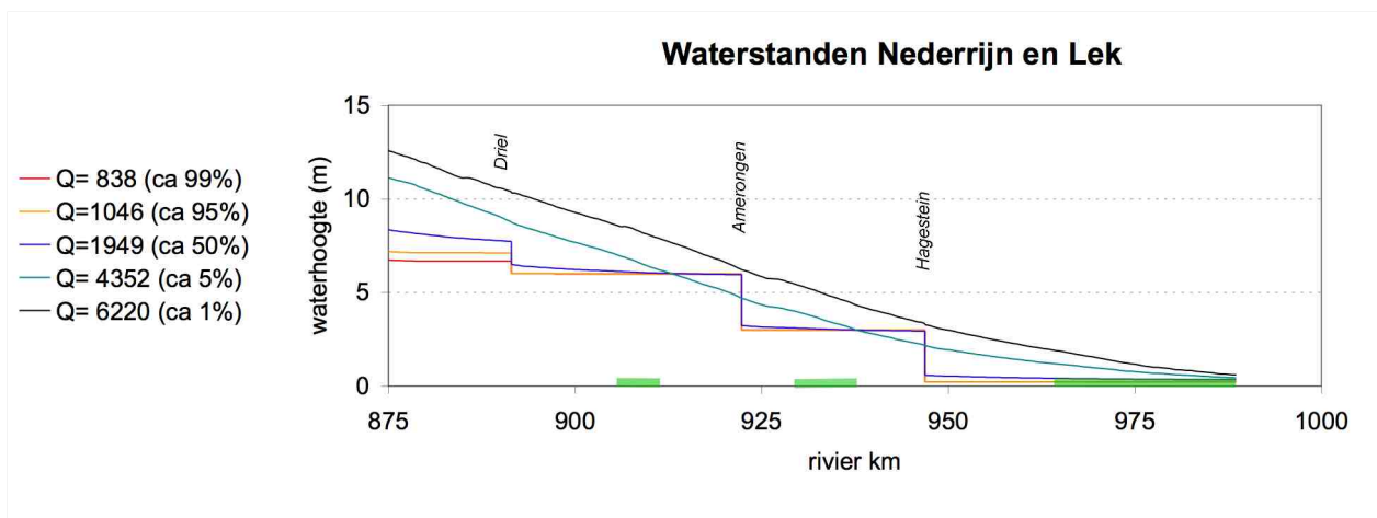
Figuur 4.2: Waterstandsverloop bij verschillende afvoeren in de Nederrijn-Lek. groene zones zijn potentieel het meest geschikt voor de groei van waterplanten omdat de waterstanden niet dalen bij het strijken van de stuwen en de stijging van de waterstand niet meer dan 1 meter is (beperkt verlies lichtdoordringing).
