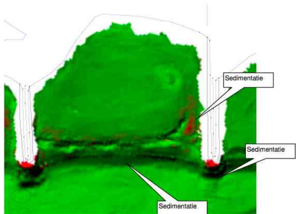
Figuur 3.4: Detailuitsnede bodemverschilkaart (2006-2012) van kribvak E. Te zien is de sedimentatiezone (donkergroen en rood) net voor en achter de vooroevers. Ook is sedimentatie rond de kribkoppen en bij de instroomopening te zien. (bron: Klarenbeek 2012).
