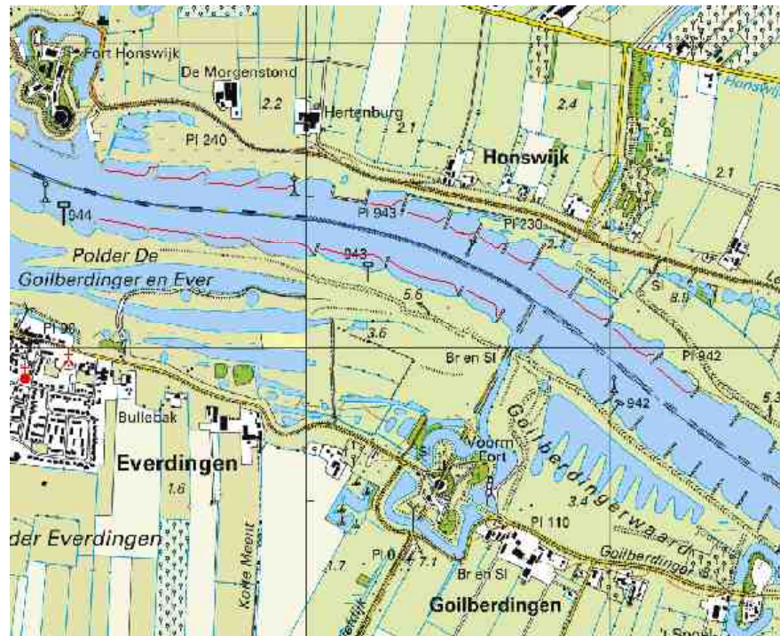
Figuur 2.4: ligging vooroevers in de Lek bij Everdingen en de Steenwaard/Honswijk. (bron: Kok in prep.).
