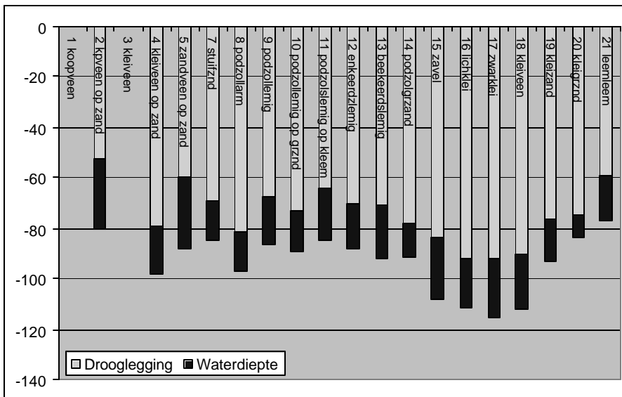
Figuur 14 Diepte en Drooglegging van het tertiaire ontwateringsysteem per bodemtype. Type 1 en 2 komen niet voor.
