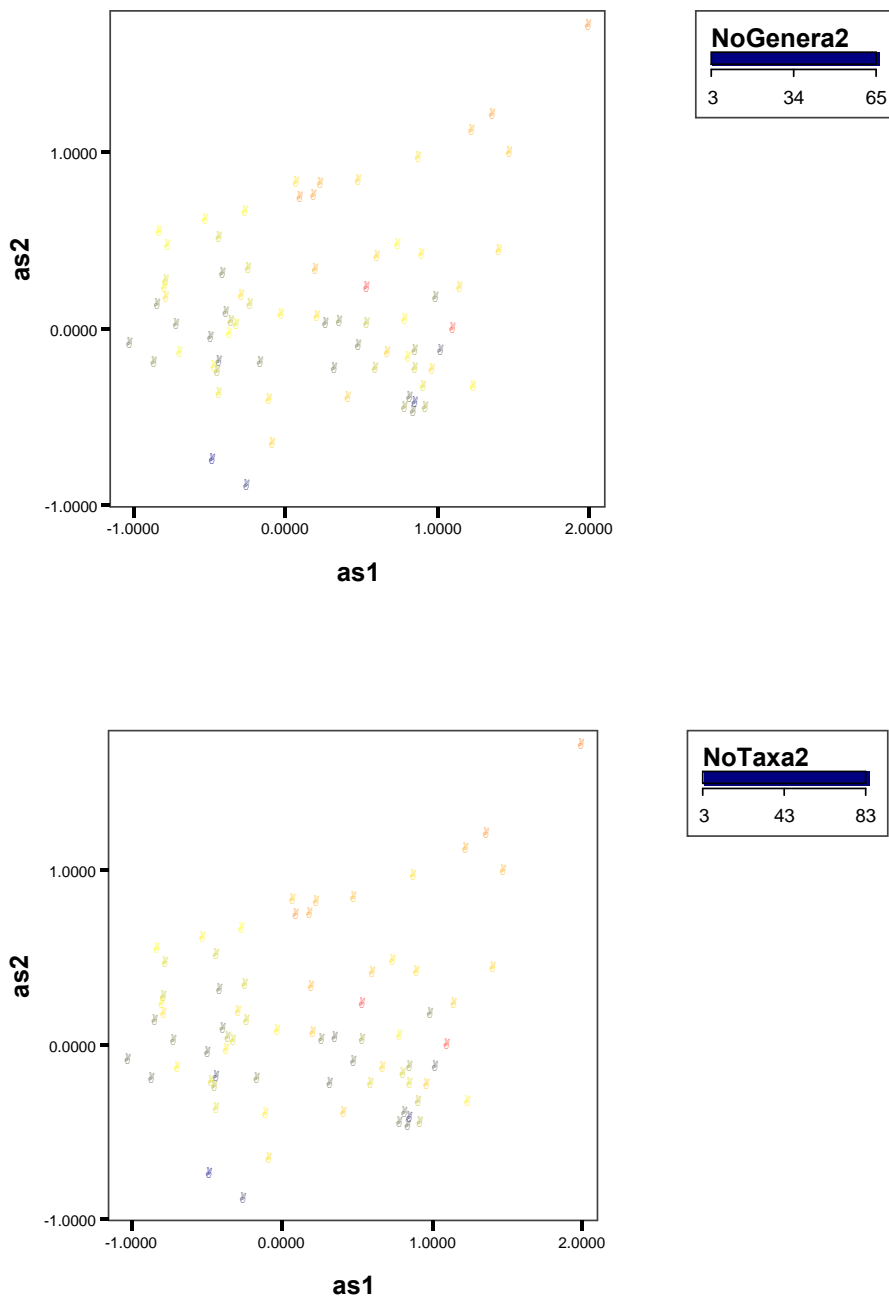
Figuur 36 Ligging monsters op de eerste en tweede ordinarie-as van de analyse waarbij alleen monsters betrokken zijn waar meerdere habitats bemonsterd zijn. Monsters zijn gelabeld met aantal genera (boven) en aantal taxa (onder). Voor de leesbaarheid van de figuur is het monster met de hoogste waarden (83 voor genera en 100 voor taxa) weggelaten).
