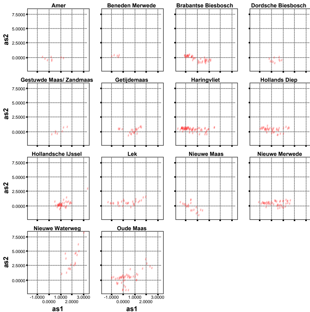
Figuur 28 Posities van de litoraal monsters op de eerste en tweede ordinatie-as van de analyse waarbij alleen de gegevens van de macrofauna zijn geanalyseerd. Per onderzocht watersysteem zijn de posities van de betrokken monsters weergegeven.
