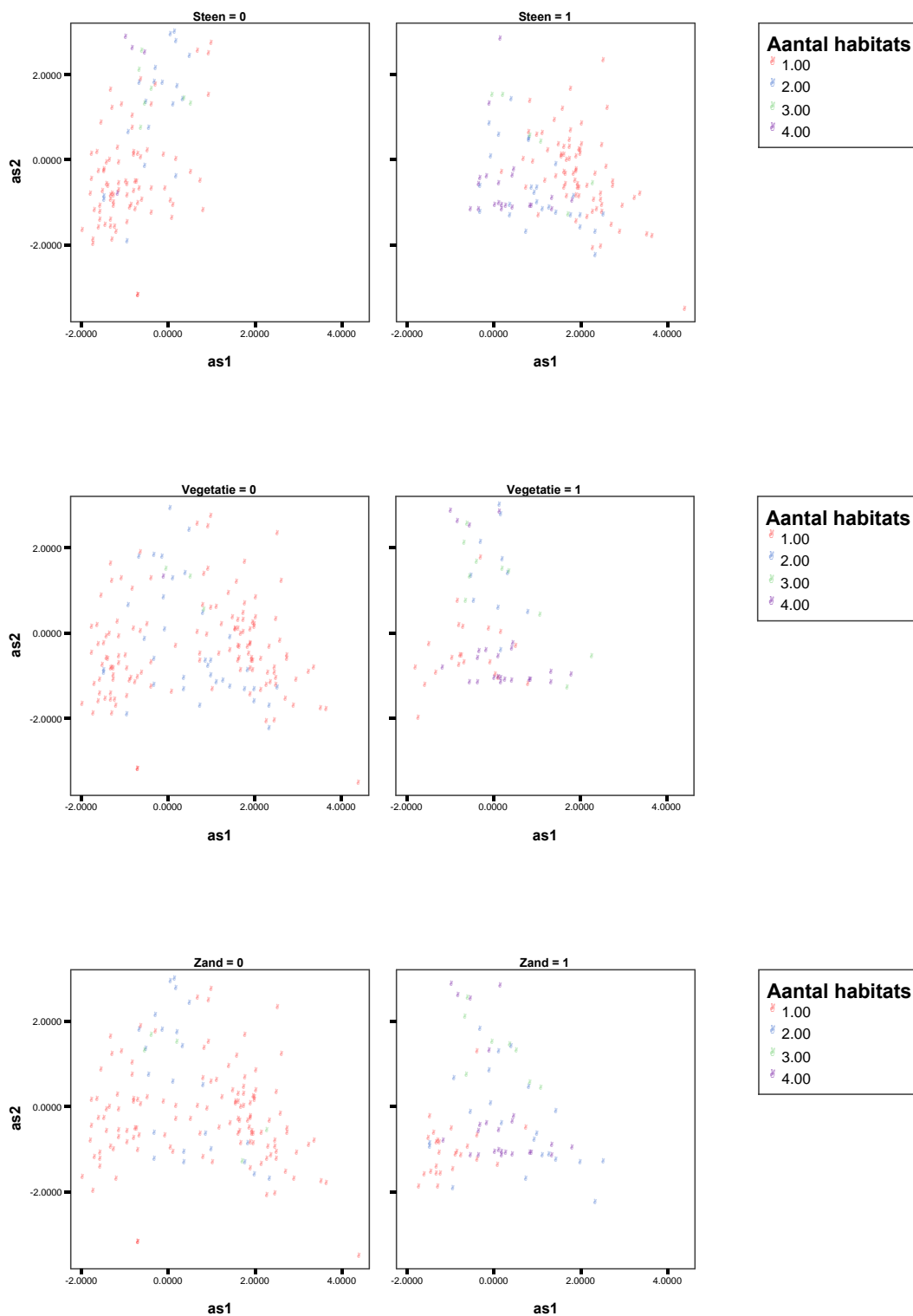
Figuur 34 Posities van de monsters voor de eerste en tweede ordinarie-as voor een directe ordinarie van de macrofauna. De monsters zijn per habitat (hout, slib, steen, vegetatie of zand) gelabeld met het aantal bemonsterde habitats. In de rechter grafiek staan steeds de monsters waar het habitat is bemonsterd, in de linker de overige monsters.
