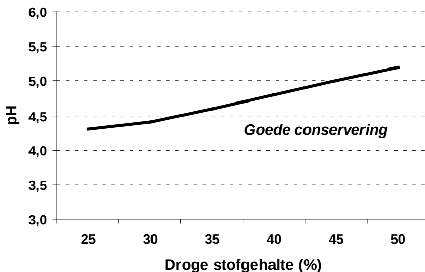
Figuur 5.2 Grenswaarden zuurgraad voor een goed geslaagde kuil bij diverse drogestofgehalten
