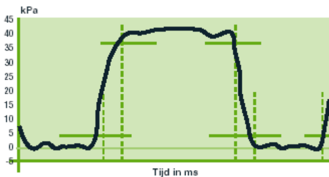
Figuur 9.2 De pulsatiecurve
