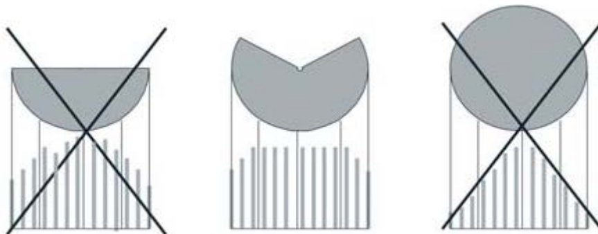
Figuur 11.4 De gewenste sectorinstelling voor een haspelinstallatie. De hoek is 240 graden. Met deze instelling wordt het beste sproeibeeld verkregen. De waterverdeling wordt aangegeven met de grijze balkjes.
