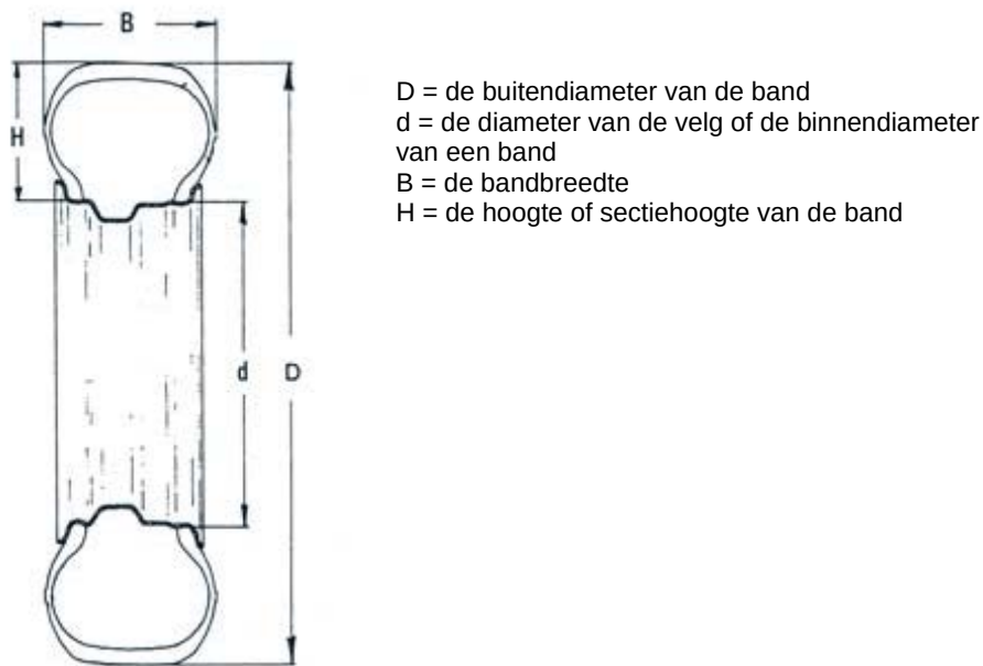
Figuur 11.2 Dwarsdoorsnede en maataanduidingen van landbouwbanden
