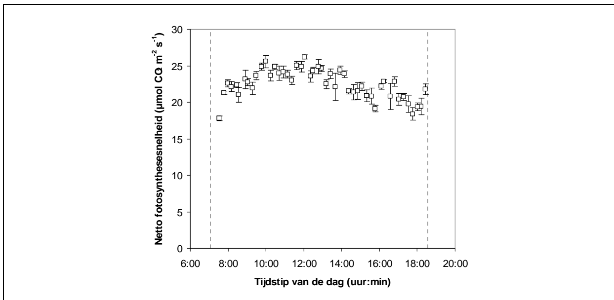
Figuur 7. Verloop van de netto fotosynthesesnelheid van tomaat gemeten bij 500 \mu\text{mol PAR m}^{-2} \text{s}^{-1} gedurende de dag. De verticale stippellijnen geven de tijdstippen van zonsopkomst en zonsondergang aan. Waarden zijn gemiddelden van 4 meetdagen begin maart 2004 \pm standaardafwijking van het gemiddelde (Bron: Dieleman en Kempkes, 2005).
