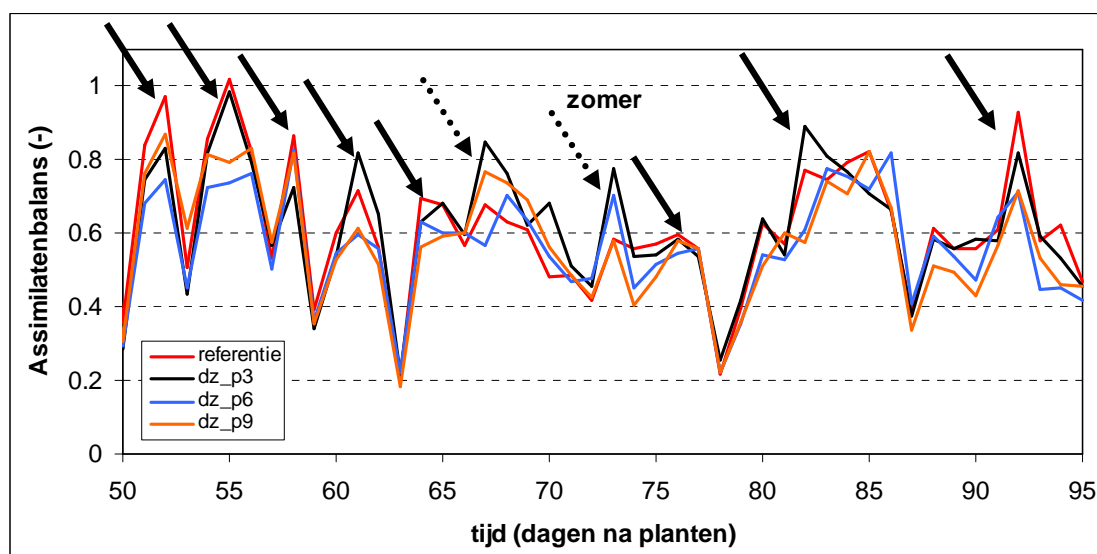
Figuur 24 Het verloop van de assimilatenbalans voor de referentieteel en de drie scenario's met verschillende dode zone in de zomer vanaf 50 dagen na planten. Een ononderbroken pijl geeft aan wanneer de assimilatenbalans in alle of de meeste scenario's werd gestabiliseerd, en een onderbroken pijl geeft aan wanneer de assimilatenbalans in alle of de meeste scenario's juist minder stabiel werd.
