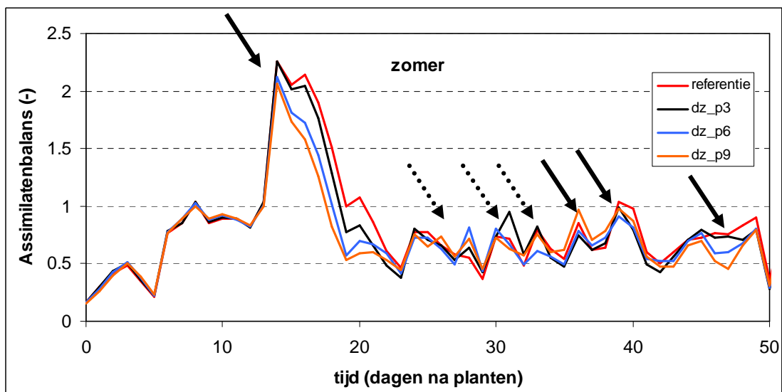
Figuur 23 Het verloop van de assimilatenbalans voor de referentieteelt en de drie scenario's met verschillende dode zone in de zomer tot 50 dagen na planten. Een ononderbroken pijl geeft aan wanneer de assimilatenbalans in alle of de meeste scenario's werd gestabiliseerd, en een onderbroken pijl geeft aan wanneer de assimilatenbalans in alle of de meeste scenario's juist minder stabiel werd.
