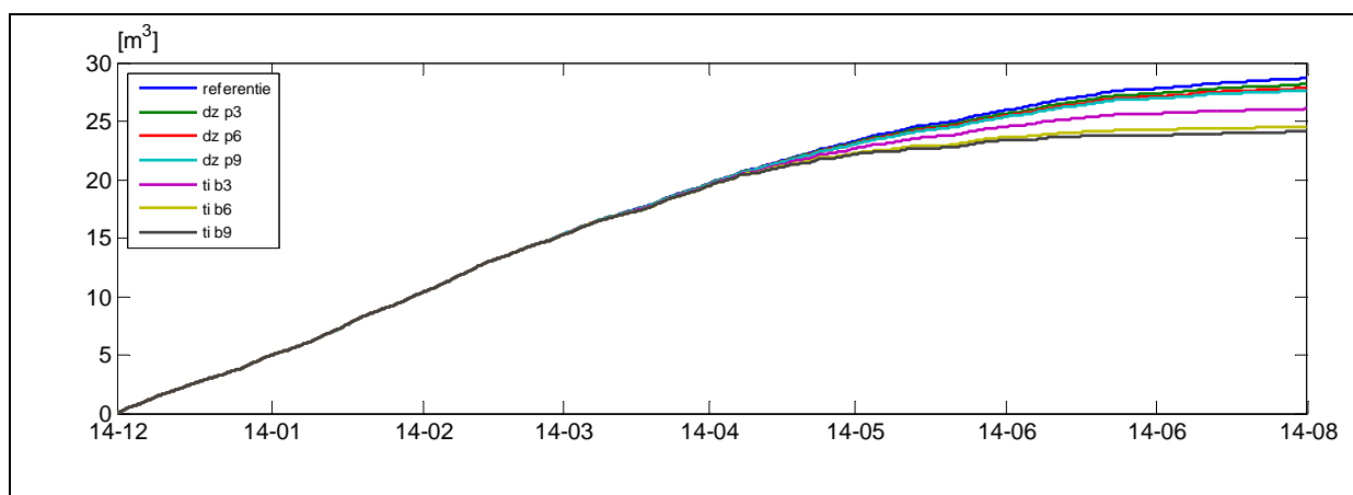
Figuur 14 Cumulatief gasgebruik voor de periode 14 december tot 14 augustus.
