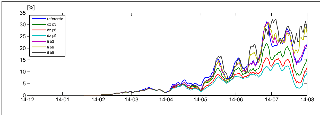
Figuur 18 Voortschrijdend gemiddelde over 7 dagen van de raamstand aan de luwe zijde.
