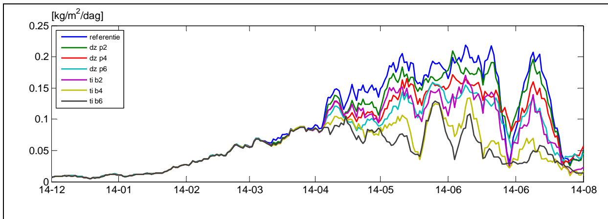
Figuur 19 Dagelijks gedoseerde totale hoeveelheid CO 2 (ketel + zuiver), een voortschrijdend gemiddelde van 7 dagen
