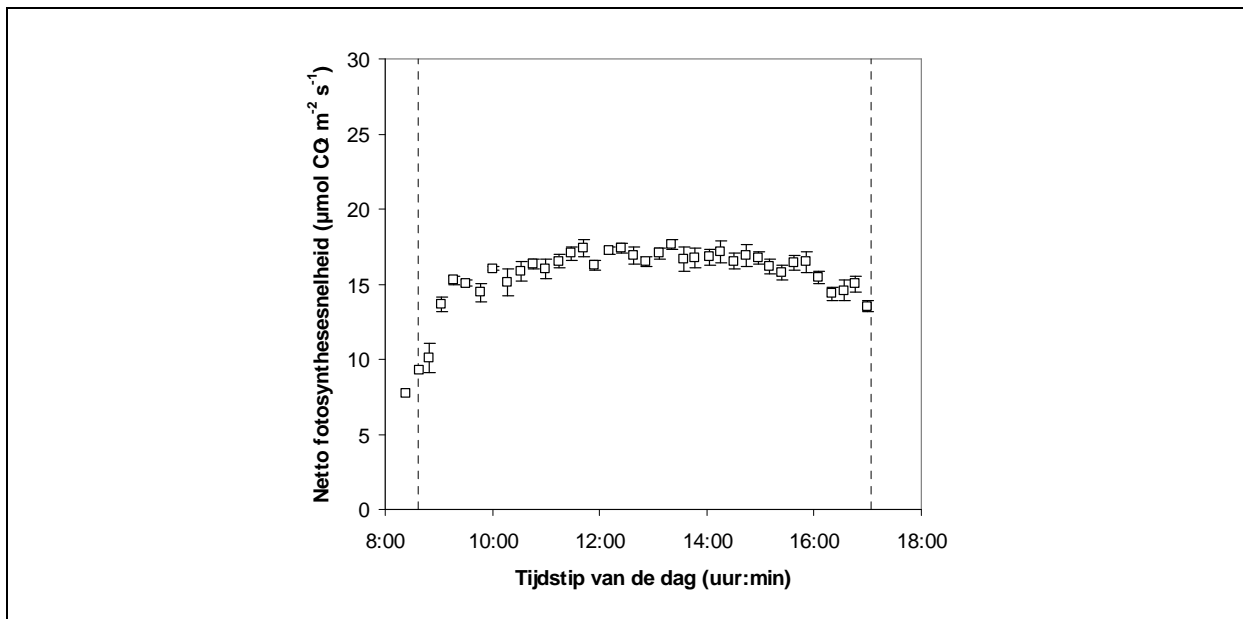
Figuur 6. Verloop van de netto fotosynthesesnelheid van tomaat gemeten bij 500 \mu\text{mol PAR m}^{-2} \text{s}^{-1} gedurende de dag. De verticale stippellijnen geven de tijdstippen van zonsopkomst en zonsondergang aan. Waarden zijn gemiddelden van 4 meetdagen in januari 2004 \pm standaardafwijking van het gemiddelde (Bron: Dieleman en Kempkes, 2005).
