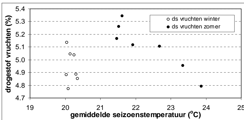
Figuur 21 Het drogestofpercentage van de vruchten in relatie tot de gemiddelde seizoenstemperatuur, in de winter- en zomerteelt, gebundeld voor de referentie en de zes cases.
