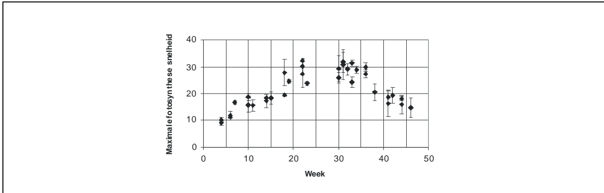
Figuur 11 Verloop van de maximale fotosynthesesnelheid (µmol CO 2 m 2 s -1 ) in de loop van het groeiseizoen 2001 voor de bovenste bladlaag van een tomatengewas (Bron: van den Boogaard & Elings, 2003).
