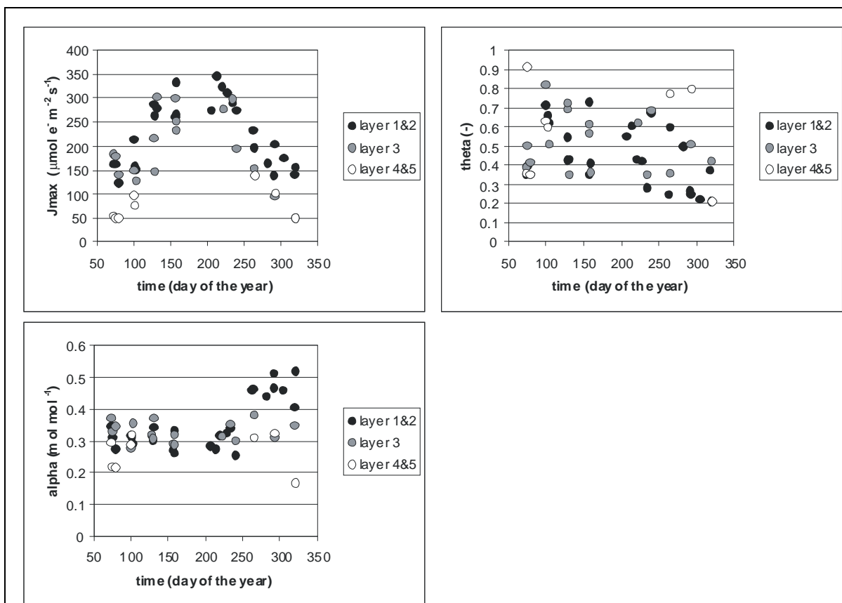
Figuur 13 Verloop van de fotosynthese-karakteristieken van tomatenbladeren van de experimenten in het voor- en najaar van 2001 in de IMAG-kas. De fotosynthesekarakteristieken betreffen de maximale elektronentransportsnelheid ( J_{max} ), de lichtbenuttingsefficiëntie ( \alpha ) en de kromming van de fotosynthesecurve ( \theta ), en zijn verkregen na calibratie met optimalisatiesoftware. De gegevens zijn weergegeven per bladlaag, waarbij lagen 1 en 2 zich bovenin het gewas bevinden, laag 3 zich halverwege het gewas bevindt, en laag 4 en 5 zich onderin bevinden. (Bron: van den Boogaard & Elings, 2003).
