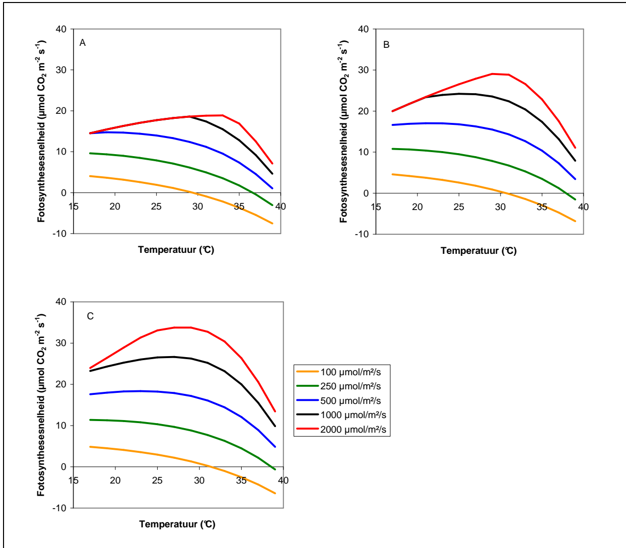
Figuur 4 Temperatuurreponscurves van de netto bladfotosynthese berekend met een gewasgroeimodel bij lichtintensiteiten oplopend van 100 naar 2000 \mu\text{mol m}^{-2} \text{ s}^{-1} en bij \text{CO}_2 concentraties van 380 ppm (A), 580 ppm (B) en 780 ppm (C) (Bron: Dieleman et al., 2003).
