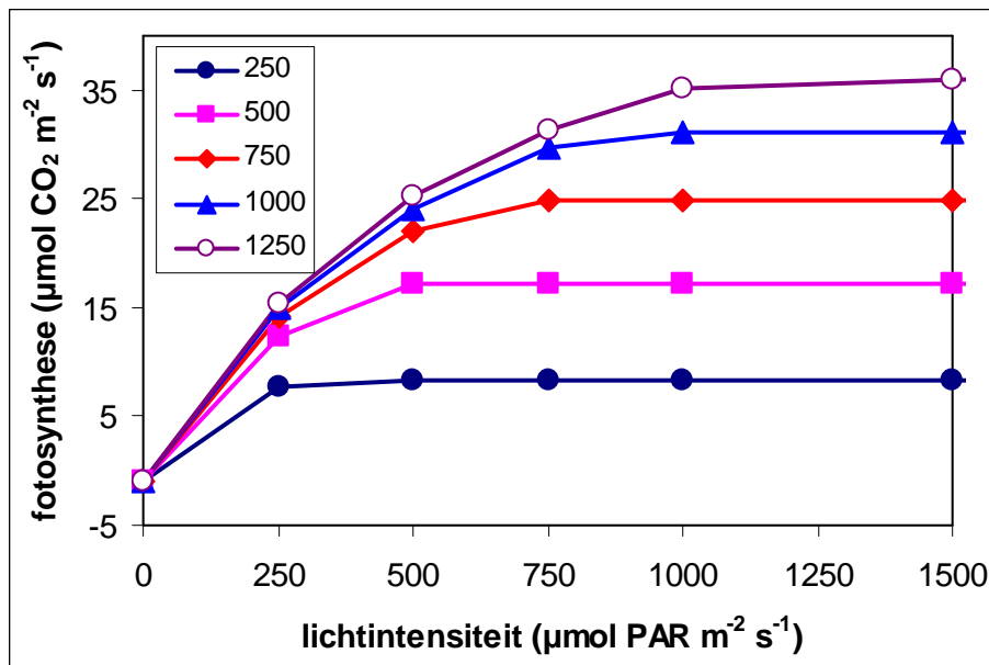
Figuur 2 Berekende lichtresponscurves van paprikabladeren bij een aantal CO 2 concentraties (zie legenda) en bij 22 °C. (Bron van uitgangsggegevens: Dieleman et al., 2003).
