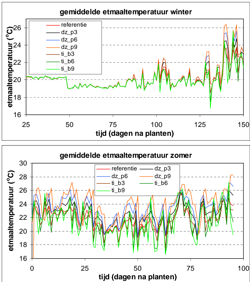
Figuur 15 Verloop van de gemiddelde etmaaltemperatuur tijdens de winter- (boven) en zomerteelt (onder) voor de referentie en de zes cases.
