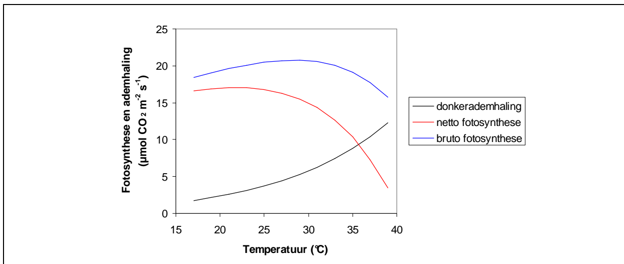
Figuur 3 Temperatuurreponscurves van de donkerademhaling, netto fotosynthesesnelheid en bruto fotosynthesesnelheid bij 500 µmol PAR m 2 s 1 en 580 ppm CO 2 berekend met een gewasgroeimodel (Bron: Dieleman et al., 2003).
