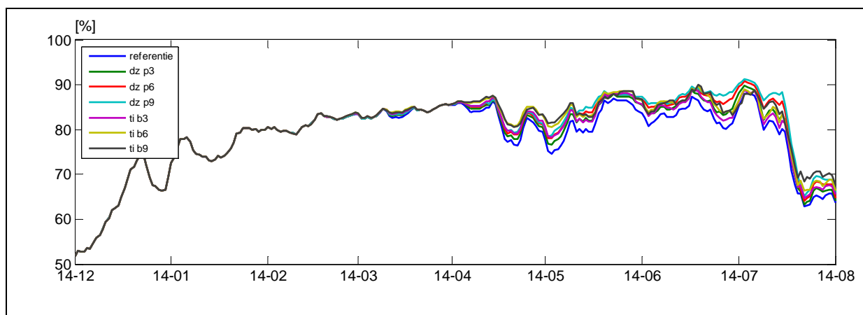
Figuur 16 Voortschrijdend gemiddelde over 7 dagen van etmaalgemiddelden van de kaslucht-RV voor de winter en zomerteelt.
