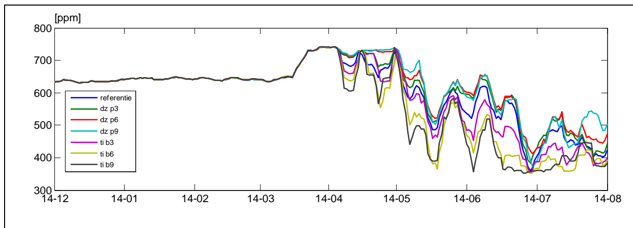
Figuur 17 Voortschrijdend gemiddelde over 7 dagen van etmaalgemiddelde CO 2 -concentratie tijdens de uren waarin gedoseerd wordt.
