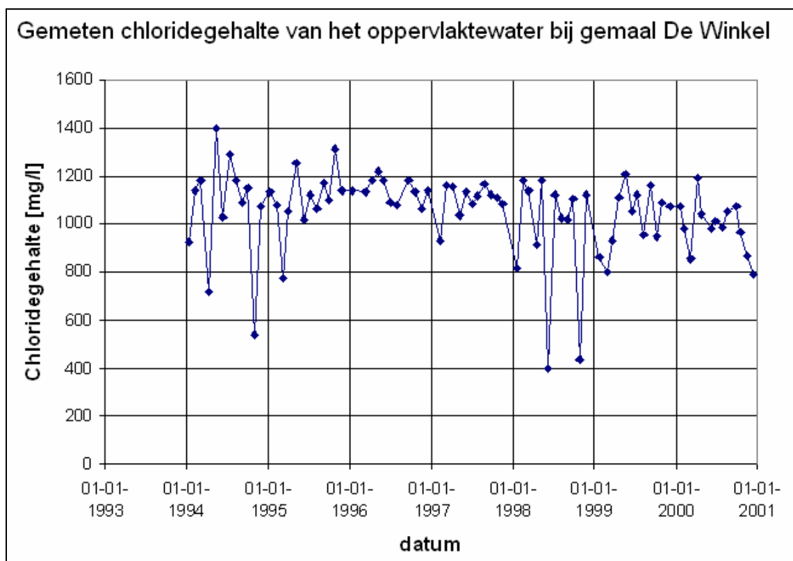
Figuur 10 Gemeten chloridegehalte van het uitgemalen water
