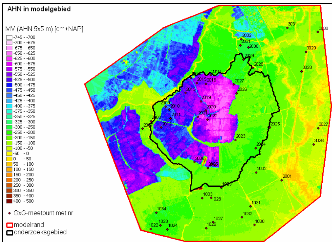
Figuur 2 Locaties van de in maart 2008 gemeten grondwaterstanden
