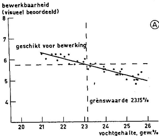
Figuur 3 Afleiding bewerkingsgrens, bewerkingstijdstip en bewerkingstraject
