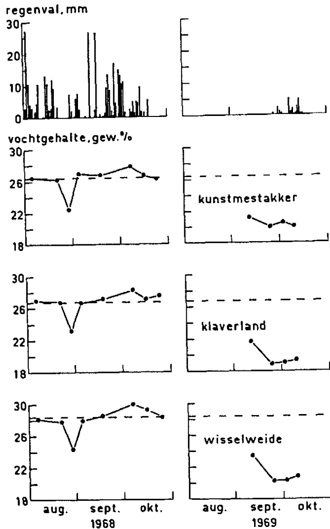
Figuur 6 Verloop van het vochtgehalte in het najaar t.o.v. de bewerkingsgrens
