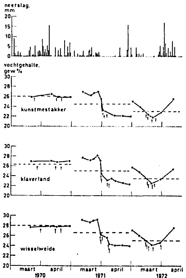
Figuur 5 Verloop van het vochtgehalte in het voorjaar t.o.v. de bewerkingsgrens:
