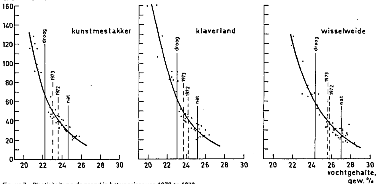
Figuur 7 Plasticiteit van de grond in het voorjaar van 1972 en 1973 1972 = gemiddelde vochtgehalte in de periode 1 maart tot 24 april 1973 = gemiddelde vochtgehalte in de periode 12 maart tot 18 april droog = gemiddelde van de vier laagste vochtgehalten nat = gemiddelde van de vier hoogste vochtgehalten
