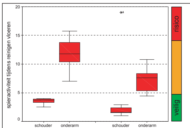
Fig. 1: Een rechte spuitlans met fingertiphandgreep vergt minder spieractiviteit in de schouder en de onderarm dan een standaardhandgreep met schuine lans.
