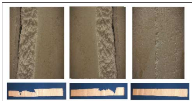
Fig. 2: Spuitbeeld van de nozzles op tempex.
