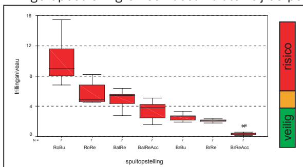
Fig. 3: Een roterende nozzle (Ro) op een gebogen lans (Bu) trilt teveel. Een rechte lans (Re) trilt minder, en ook een accumulator (Acc) is effectief. Een opstelling met breedstraalnozzle (Br) en accumulator trilt niet.
