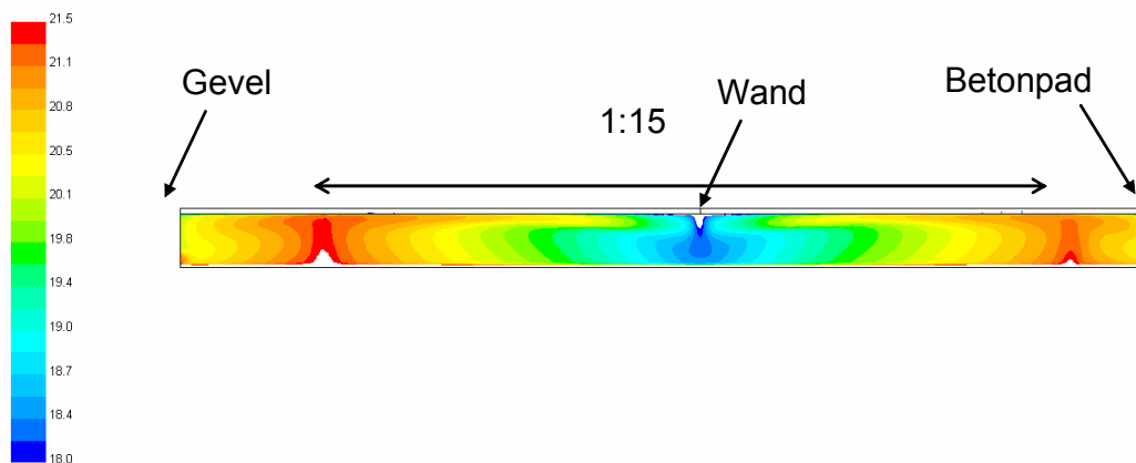
Figuur 5. Temperatuurverdeling.
