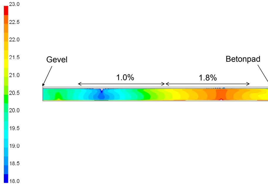
Figuur 7. Temperatuurverdeling.
