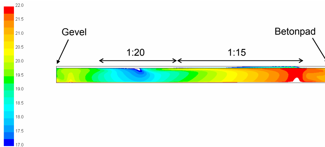
Figuur 4. Temperatuurverdeling.
