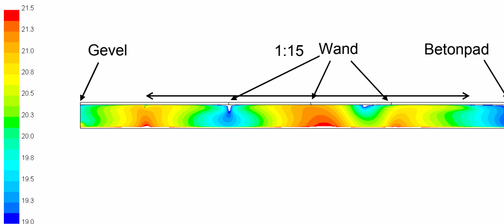
Figuur 6. Temperatuurverdeling.
