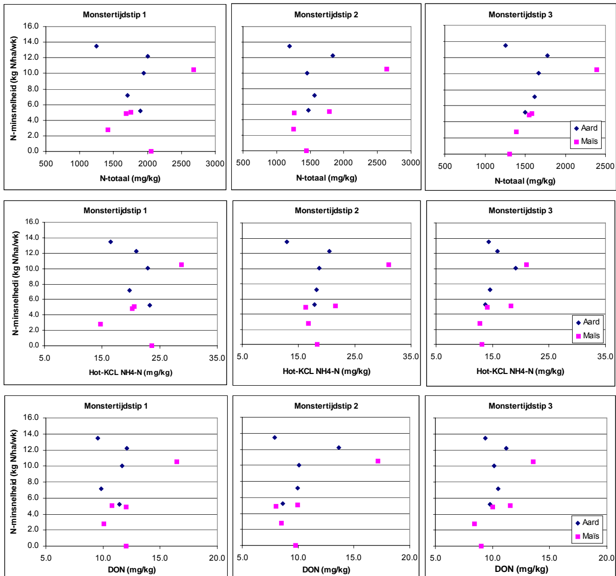
Figuur 11 Relaties mineralisatiesnelheid en bodemparameters N-totaal, Hot KCL NH4-N en DON (laag 0-30 cm) op bemonsteringstijdstip 1 (27 maart), 2 (4 april) en 3 (21 april) van de braakvelden per gewasplot
