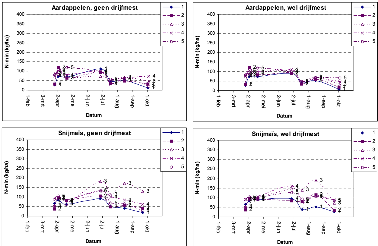
Figuur 15 Verloop N-mineraal (laag 30-60 cm) van de N0-behandeling per blok (1t/m 5) voor aardappelen en snijmais, met en zonder drijfmest
