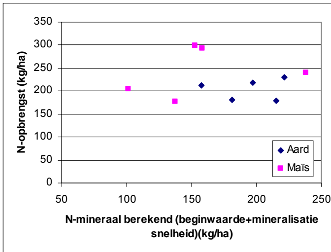
Figuur 19 Relatie tussen berekende hoeveelheid N-mineraal in de laag 0-30 cm in het groeiseizoen rond 1 juli en N-opbrengst van aardappelen en snijmais op de velden zonder bemesting
