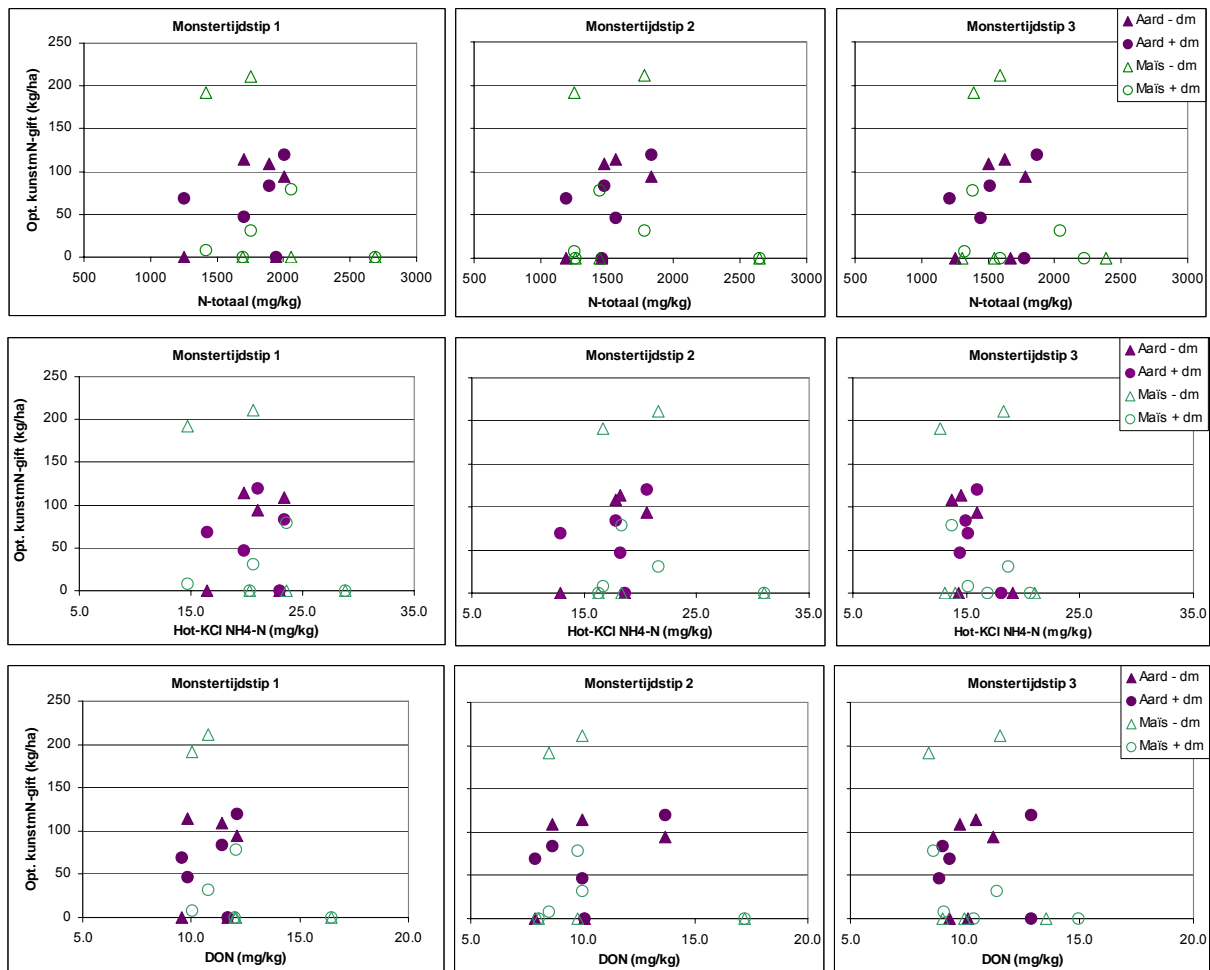
Figuur 9 Relaties optimale kunstmest-N-gift met de bodemparameters N-totaal, Hot KCL NH 4 -N en DON, laag 0-30 cm op bemestingstijdstip 1 (27 maart), 2 (4 april) en 3 (21 april) voor de gewassen aardappelen en snijmaïs, met (+ dm) en zonder (- dm) drijfmest
