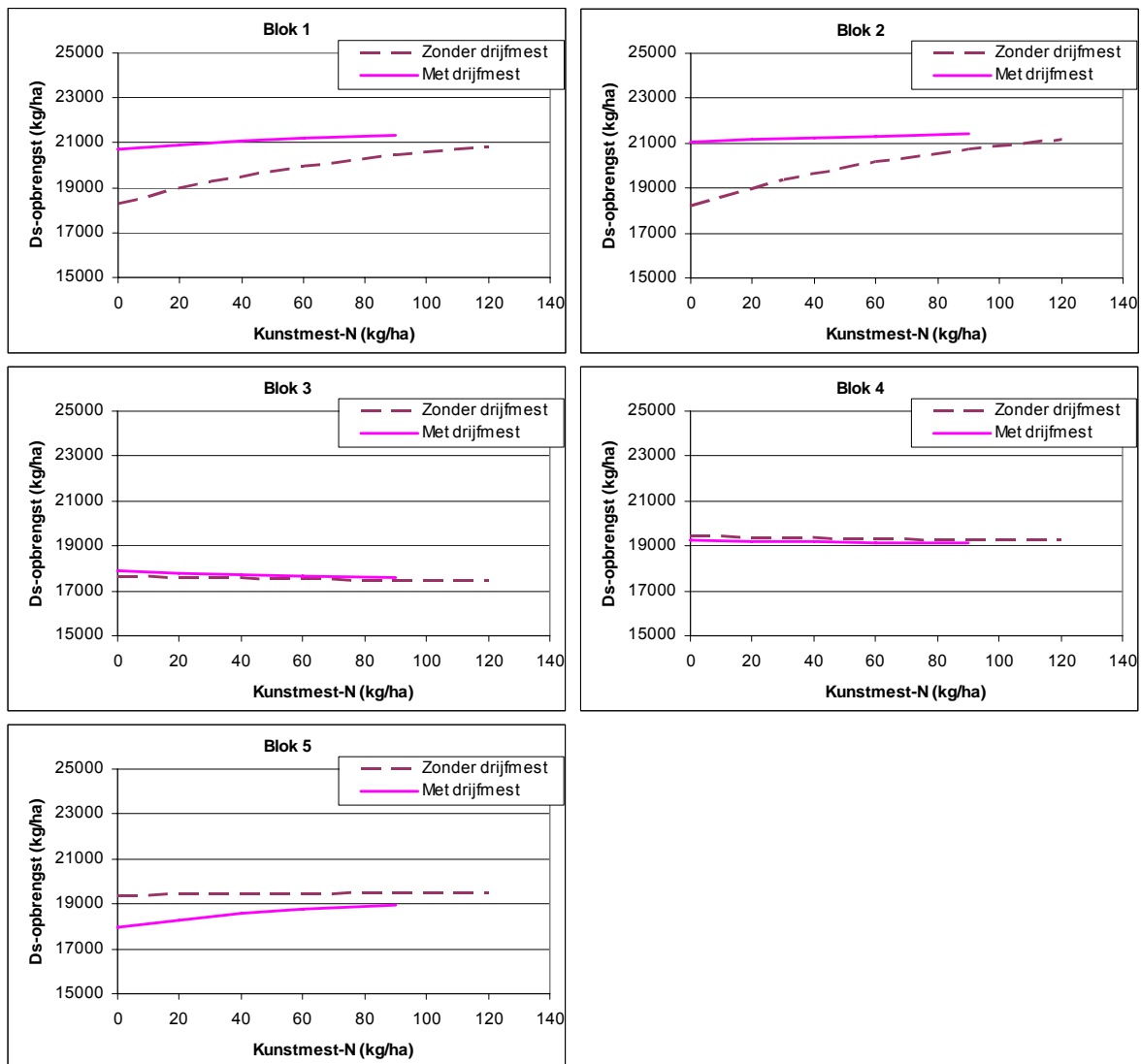
Figuur 6 Gemodelleerde relatie tussen drogestofopbrengst en N-kunstmestgift per blok voor het gewas snijmais bij de behandelingen zonder (-dm) en met (+dm) drijfmest
