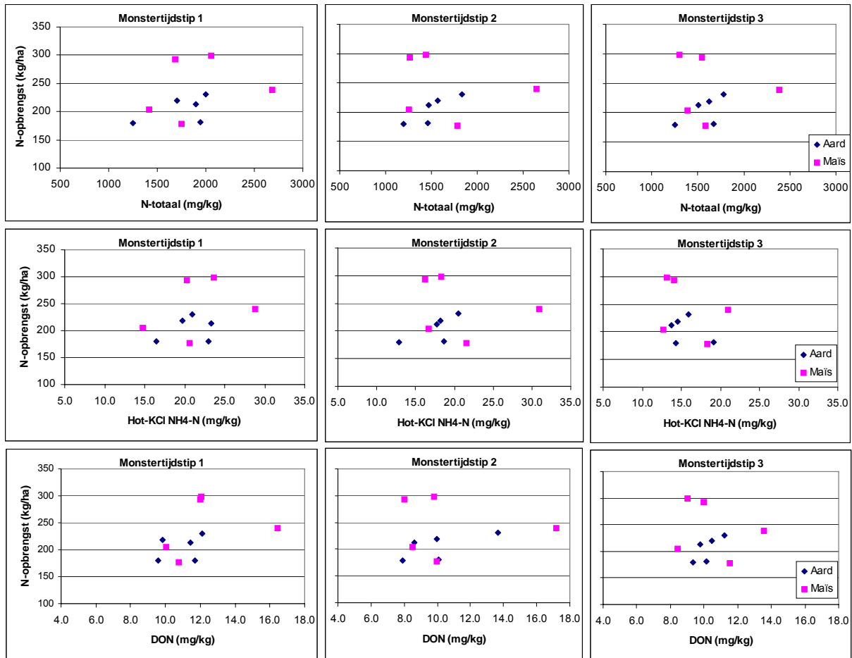
Figuur 10 Relaties stikstof opbrengsten van de NO-velden met de bodemparameters N-totaal, Hot KCL NH4-N en DON, laag 0-30 cm op bemonsteringstijdstip 1 (27 maart), 2 (4 april) en 3 (21 april) voor de gewassen aardappelen en snijmaïs
