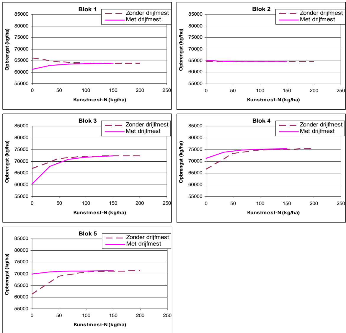
Figuur 5 Gemodelleerde relatie tussen vermarktbare opbrengst en kunstmest-N gift per blok voor het gewas aardappelen bij de behandelingen zonder en met drijfmest
