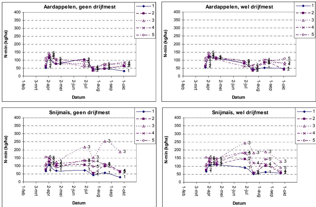
Figuur 4 Verloop N-mineraal (laag 0-30 cm) van de NO-behandeling per blok (1t/m 5) voor aardappelen en snijmaïs, met en zonder drijfmest
