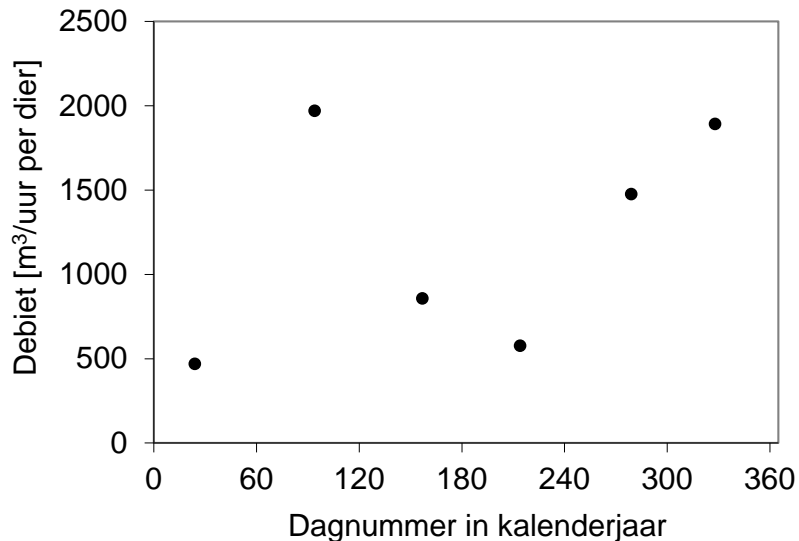
Figuur 4 Gemiddelde ventilatie-debiet [ \text{m}^3/\text{uur} per dier] op alle verschillende meetdagen
