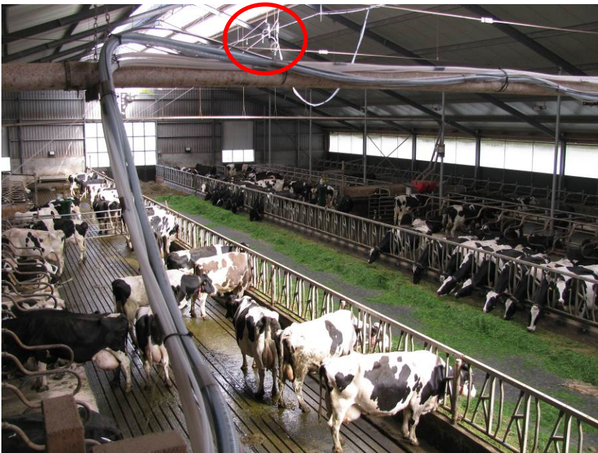
Twee cyclonen (PM10 en PM2,5) voor de bepaling van fijn stof in de luchtstroming van de uitgaande lucht.
