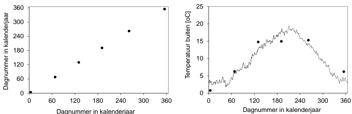
Figuur 4 Verdeling van de metingen over het jaar (a), en de buitentemperatuur (b) vergeleken met de gemiddelde waarden gemeten over de jaren 1991-2010 bij het KNMI-weerstation Leeuwarden ( www.knmi.nl ; als stippelijijn weergegeven).
