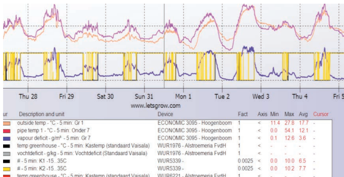
Figuur 9. Verloop van buitentemperatuur, inzet van de LBK, kastemperatuur en VD in de periode tussen 27-07 en 05-08-2011.
