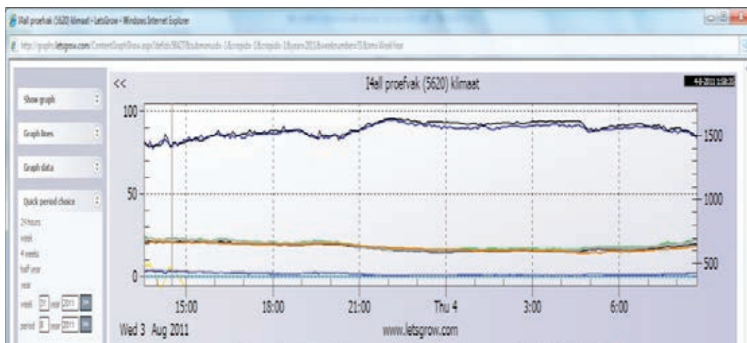
Figuur 3. Verloop van kasttemperatuur en RV tijdens moment B gemeten door de meetpalen.
