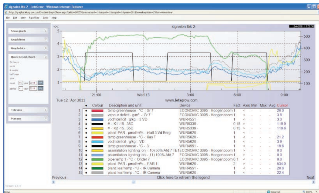
Figuur 1. Close up op Vochtdeficit, ventilatorstand en buistemtemperatuur in de nacht van 12-4-2011.
