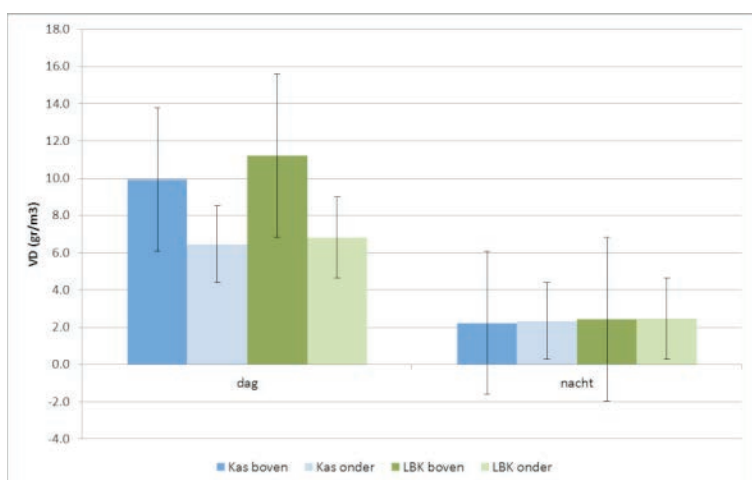
Figuur 14. Gemiddeld VD in proefvak (LBK) en referentie (kas) en op kophoogte (boven) en tussen het gewas (onder) over de dagen 01-08-2011 tot 07-08-2011 (gem. etmaaltemp). 19^\circ\text{C} ).
