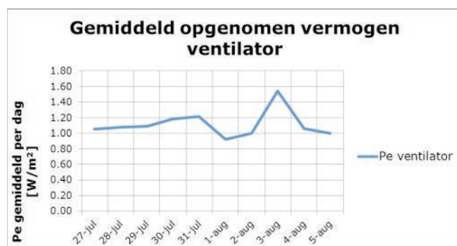
Figuur 10. Gemiddeld opgenomen energie van de ventilator in W/m².
