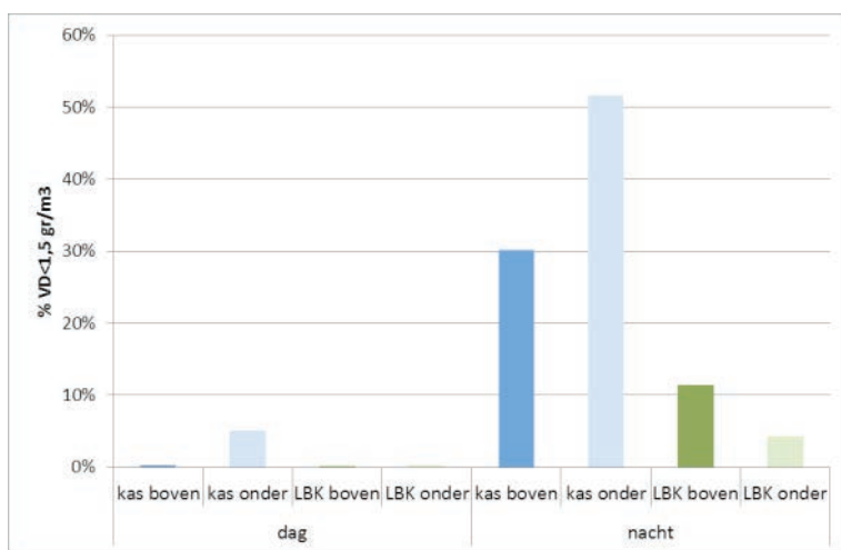
Figuur 17. % van totaal metingen dat VD < 1,5 \text{ gr/m}^3 in proefvak (LBK) en referentie (kas) en op kophoogte (boven) en tussen het gewas (onder) over de dagen 21-07-2011 tot 31-07-2011 (gem. etmaaltemp). 16 °C).
