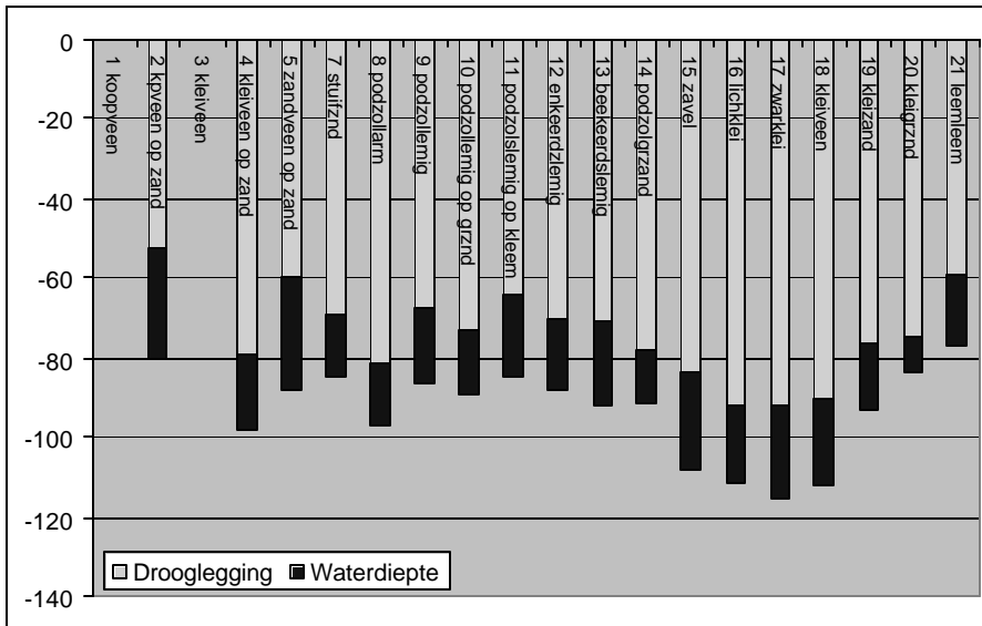
Figuur 14 Diepte en Drooglegging van het tertiaire ontwateringsysteem per bodemtype. Type en 3 komen niet voor.
