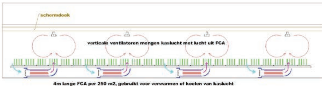
Figuur 2.2. Principe FCA systeem voor gesloten kas.
