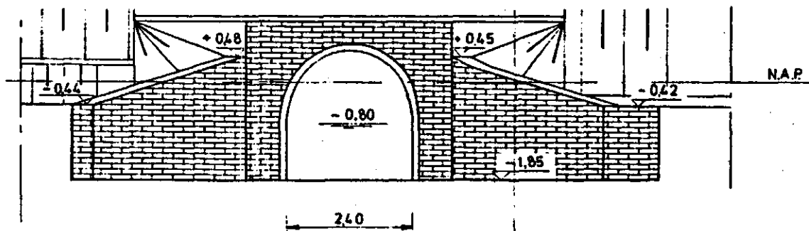
aanzicht landzijde
