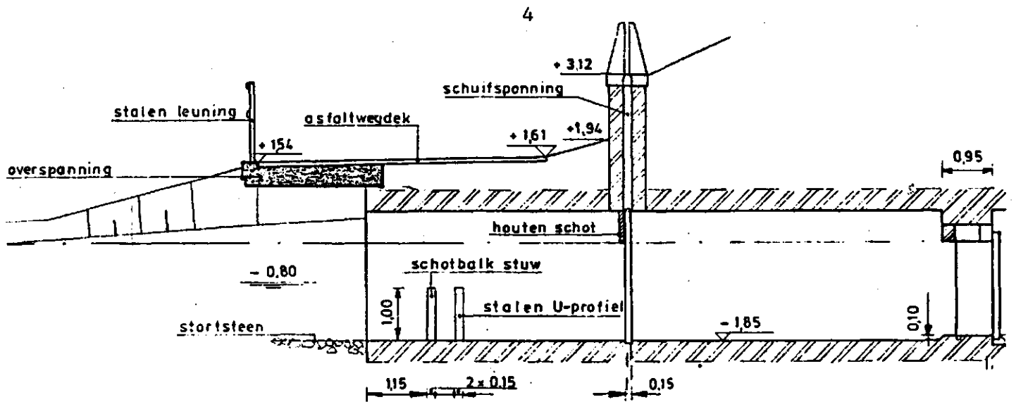
lengte doorsnede
