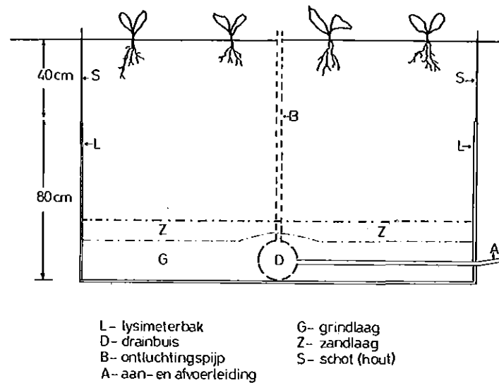
Fig. 2. Dwarsdoorsnede van de lysimeterbak
