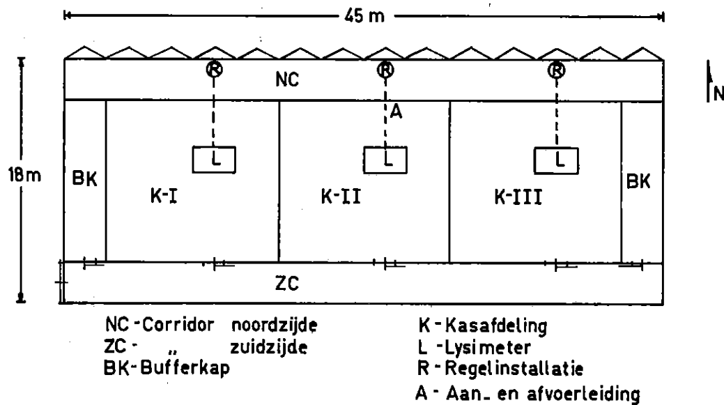
Fig. 1. Plattegrond van de lysimeterkas
