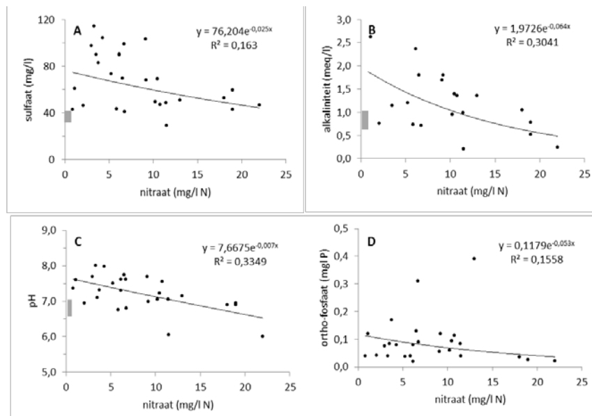
Figuur 4.4. Relaties tussen de nitraatconcentratie en enkele andere chemische variabelen van de wateren van type 13 (bronbeken). De grijze vakjes zijn de concentratiebereiken van drie (alkaliniteit, sulfaat) of vijf (pH, nitraat) Twentse bronbeken in 1957 (Maas 1959).
