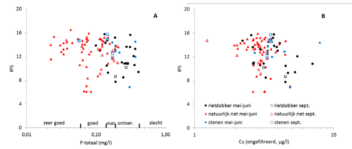
Figuur 4.6. Relaties tussen IPS en totaal-fosfaat (A) en koper (B) voor de watertypen uit de grote rivieren (R16, R07, R08, R08!) onderverdeeld naar bemonsteringsmaand en substraat. Grenzen van de kwaliteitsklassen volgens Van der Molen & Pot (2007).
