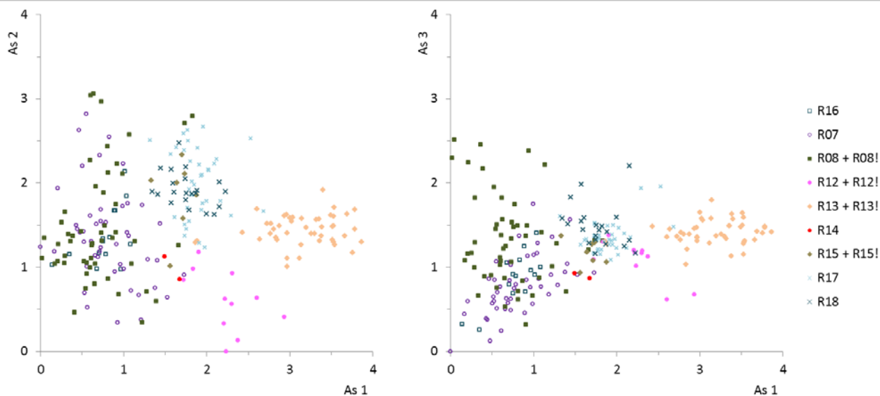
Figuur 4.3. Scores van alle fyto-benthosmonsters in een DCA-ordinatie op de eerste en tweede as (links) en eerste en derde as (rechts). De cumulatieve verklaarde variantie op de assen 1, 2 en 3 bedraagt respectievelijk 9,7, 13,9 en 17,5 procent.
