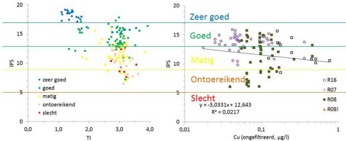
Figuur 4.8 Vergelijking van voorgestelde kwaliteitsklassen voor het fyto-benthos van de Nederlandse typen R16, R07 en R08 (rechts) met de door de overige lidstaten toegekende kwaliteitsklassen van andere zeer grote rivieren van het intercalibratietype Very Large Rivers (links).
