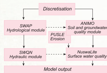
Figuur 1. Schematische weergaven van het modelinstrumentarium NL-CAT
