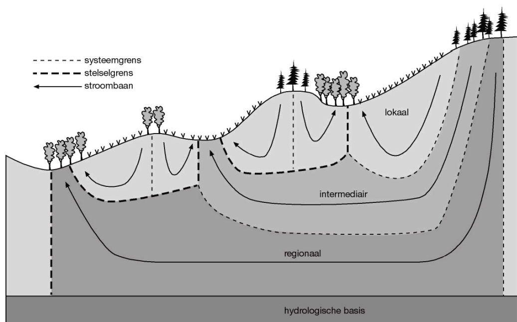
Figuur 1. Schematische weergave van lokale, intermediaire en regionale grondwatersystemen en -systeemstelsels (bron: Stuurman en Griffioen, 2003 7 ).
