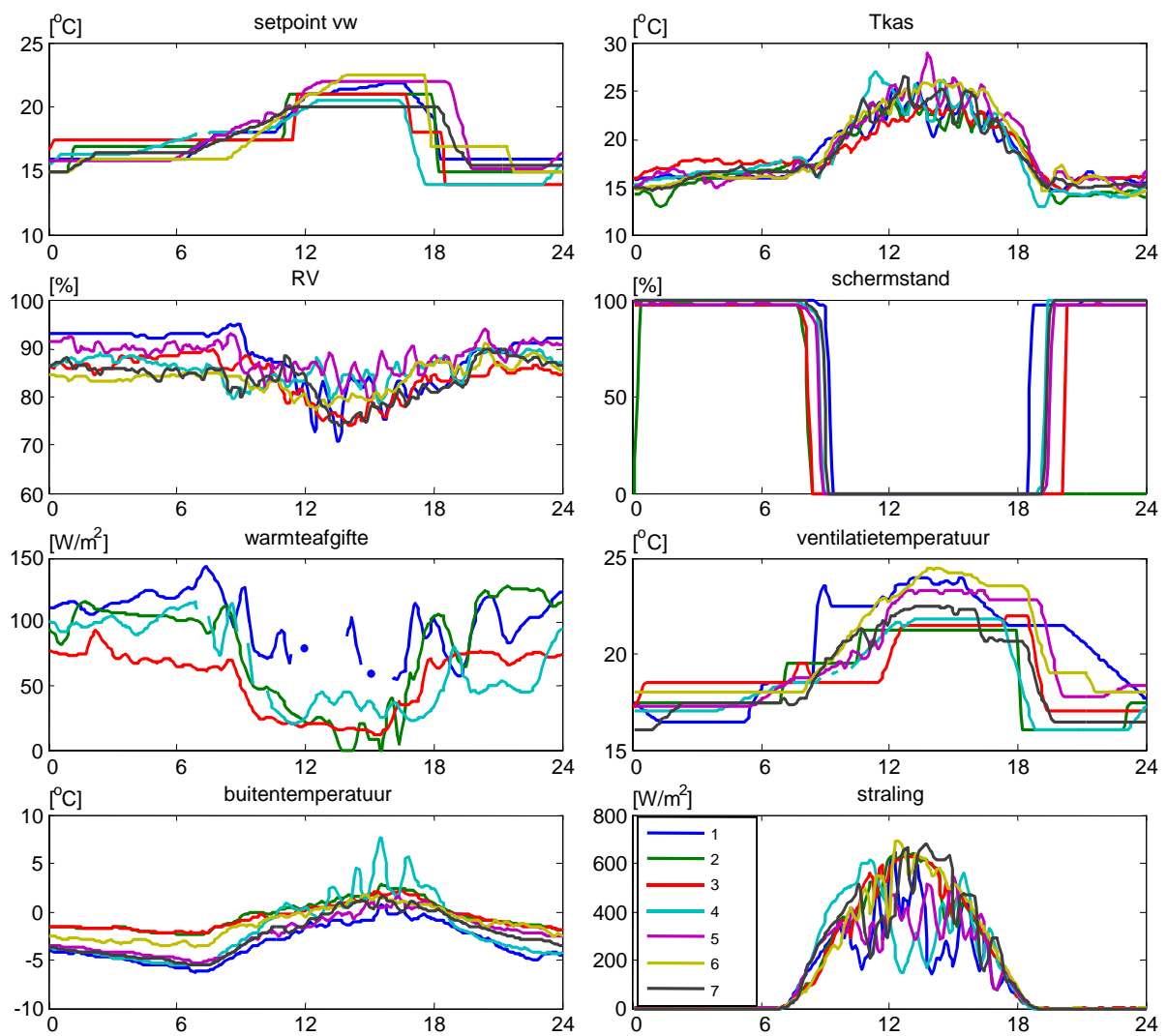
Figuur 2.3 Overzicht klimaatparameters van 12 maart 2006 (tomatenbedrijf 1 t/m 7)
