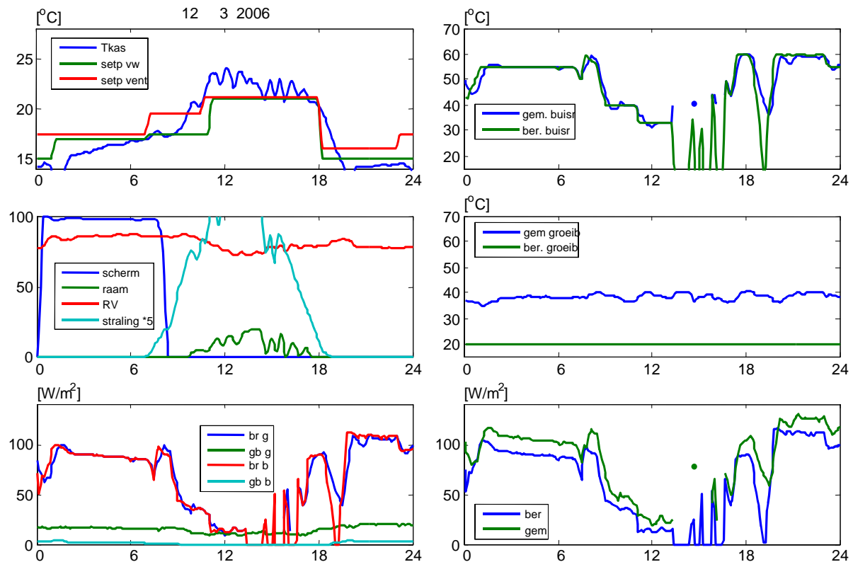
Figuur 2.4 Overzicht klimaatparameters van tomatenbedrijf 2 op 12 maart 2006
