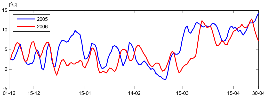
Figuur 2.5 Etmaalgemiddelde buitentemperatuur (voortschrijdend gemiddelde van 4 dagen)
