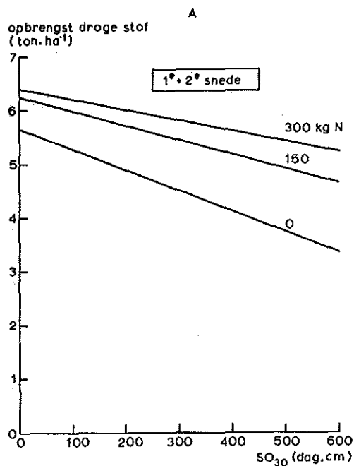
Fig. 9A. Opbrengst droge stof 1e + 2e snede van gras op veen over 1970-74 te Bleskensgraaf in relatie tot de som van overschrijdingen van de grondwaterstand gedurende november-mei ( SO_{30} ) bij stikstofgiften van 0, 150 en 300 kg.ha -1
