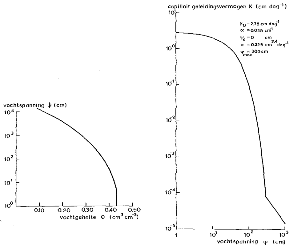
Fig. 3. Relaties tussen vochtspanning en vochtgehalte en tussen het capillair geleidingsvermogen en de vochtspanning van de zware zavelgrond
