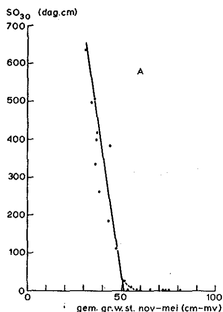
Fig. 10A. Relatie SO_{30} en de gemiddelde grondwaterstand van november-mei voor de veengrond te Bleskensgraaf
