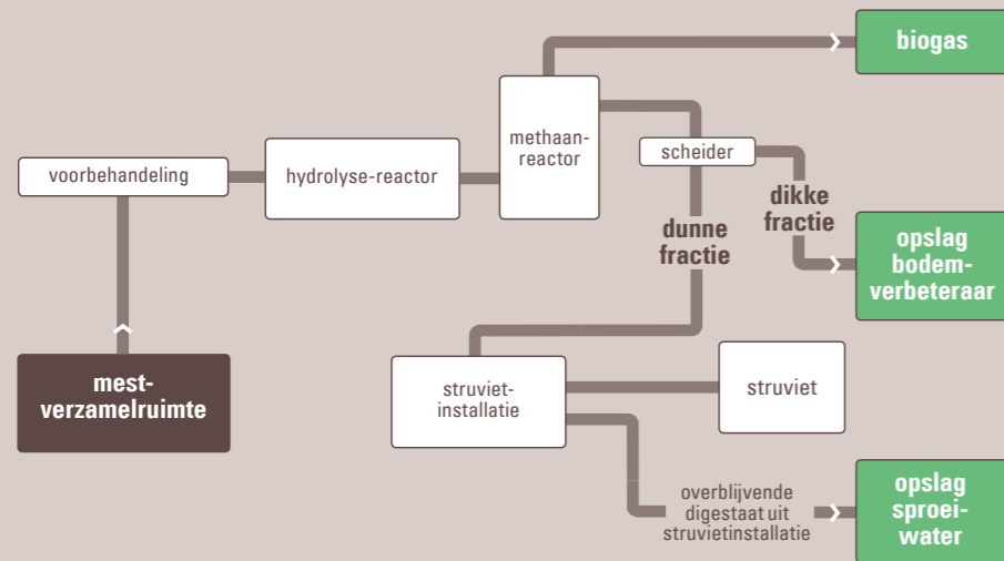
Figuur 1 – Stroomschema mestraffinage op De Marke (bron: Fermtech Systems bv)
