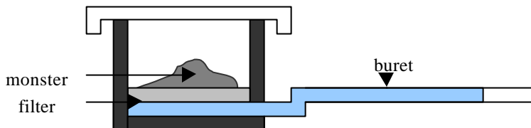
Fig. 4 Principe opstelling voor bepaling van de potentiële zwelcapaciteit
