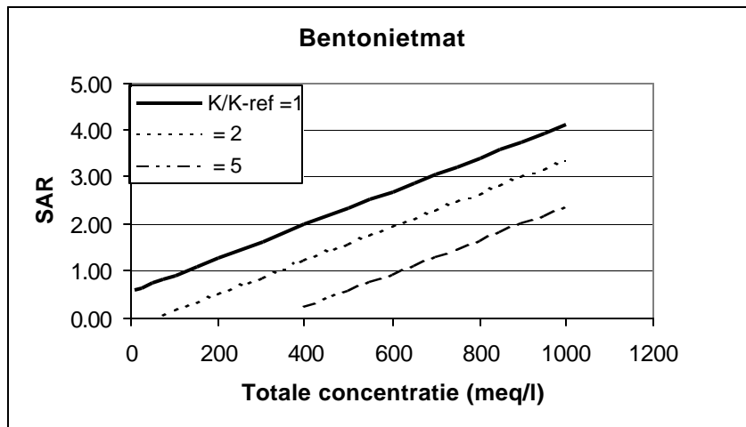
Fig. 11 C Berekende samenhang voor bentonietmat tussen totale concentratie en SAR voor enkele verhoudingen tussen actuele en referentiedoortlatendheid ( K/K\text{-ref} )
