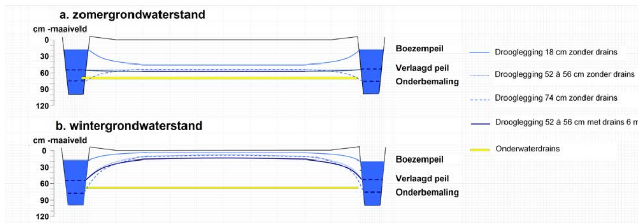
Figuur 21 Schematische dwarsdoorsnede van een perceel met a) de laagste zomergrondwaterstand voor een 'compromispeil' van 35 cm -mv en voor een hoog peil van 15 à 20 cm -mv en met b) de hoogste wintergrondwaterstand een 'compromispeil' van 35 cm en voor een lager peil van 50 à 55 cm -mv uit het onderzoek in polder Zeevang
