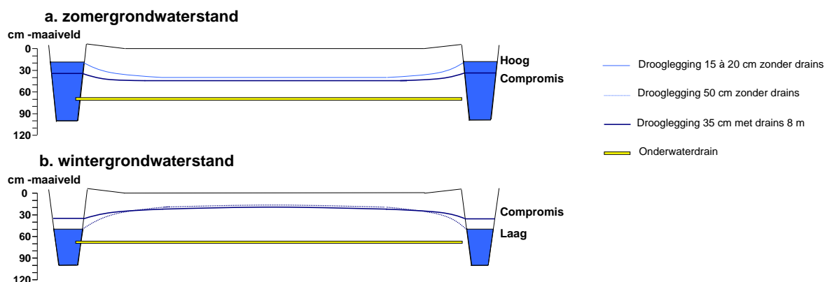
Figuur 20 Schematische dwarsdoorsnede van een perceel met a) de laagste zomergrondwaterstand voor een 'compromispeil' van 35 cm -mv en voor een hoog peil van 15 à 20 cm -mv en met b) de hoogste wintergrondwaterstand een 'compromispeil' van 35 cm en voor een lager peil van 50 à 55 cm -mv uit onderzoek op Praktijkcentrum Zegveld (Hoving et al., 2008)
