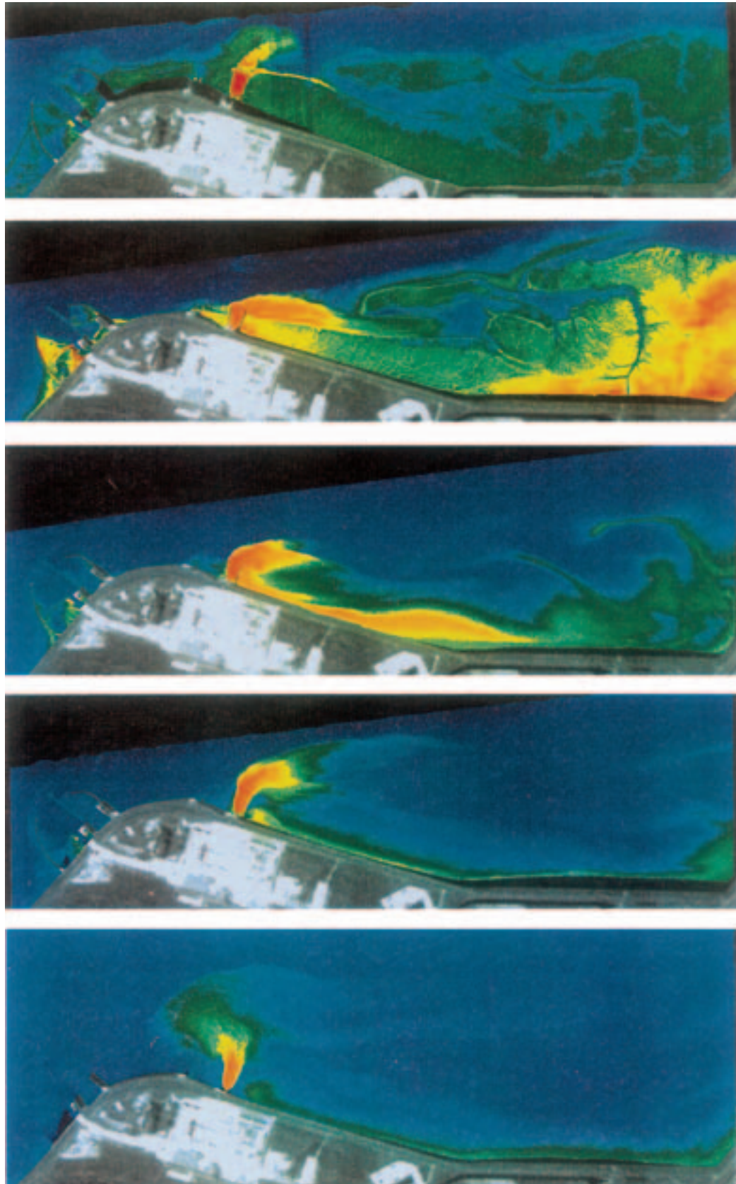
Bijlage 1: Warmtelozingsbeeld Eemscentrale tijdens verschillende momenten van de getijcyclus (Fraikin & van den Berghs, 1996).
