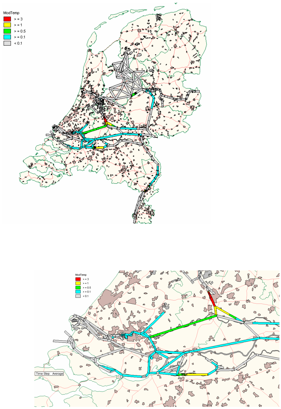
Figuur 4.4 Verskil tussen de berekende surplustemperatuur van de basisberekening (gemiddeld) en het scenario met laag Rijn- en Maasdebiet.
