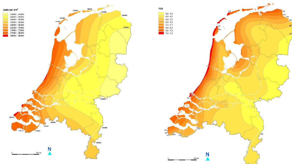
Figuur 3.2a en b. Globale straling in \text{J}/\text{cm}^2 -dagwaarden (links) en gemiddelde windsnelheid in \text{m}/\text{s} (rechts) uit KNMI klimaat-atlas ( www.knmi.nl/voorl ).
