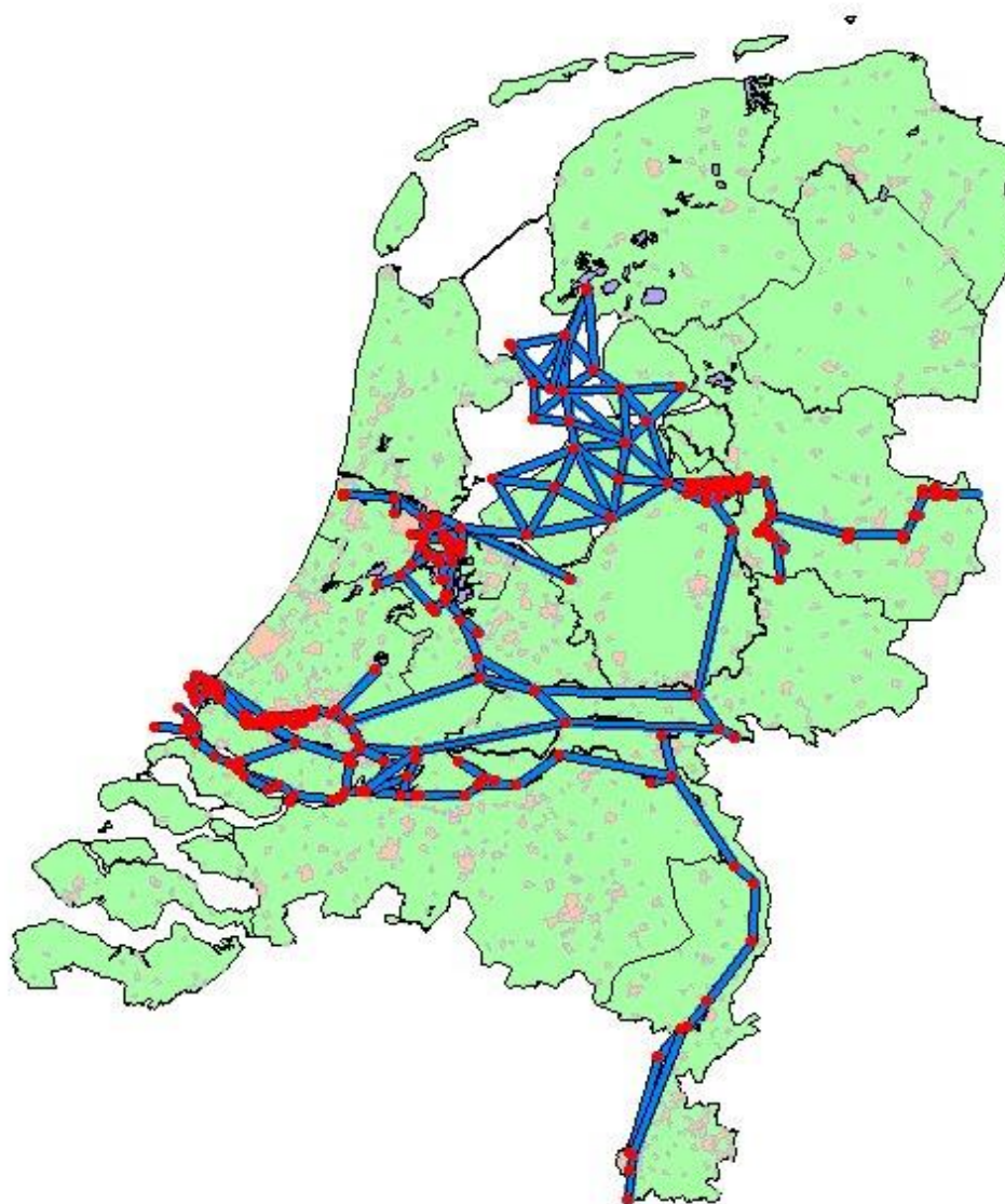
Figuur 3.1a Schematisatie van het Landelijk Temperatuurmodel in GIS met afzonderlijke kaartlagen voor kopen en takken
