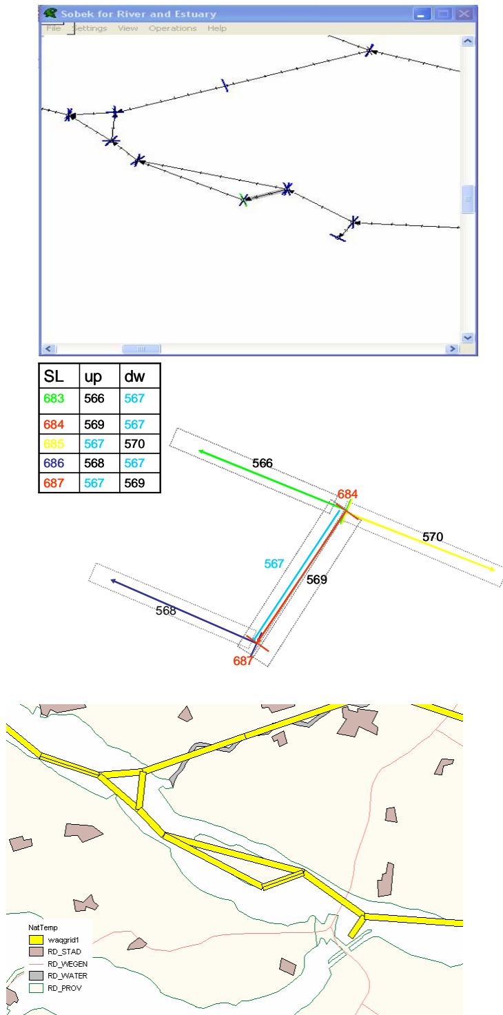
Figuur 3.8. Detail van de schematisatie rondom tak HAVL053 in het Haringvliet: (a) in SOBEK Userinterface, (b) dezelfde situatie schematisch en (3) situatie in Mapper (mbv SobRiv2Map).
