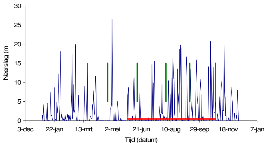
Figuur 2. De dagelijkse neerslag gemeten in Rotterdam voor de periode van de proef in 2010. Groene verticale lijnen geven aan wanneer bodemonsters zijn genomen, en de rode horizontale lijn geeft aan in welke periode de kool heeft gegroeid in het veld.
