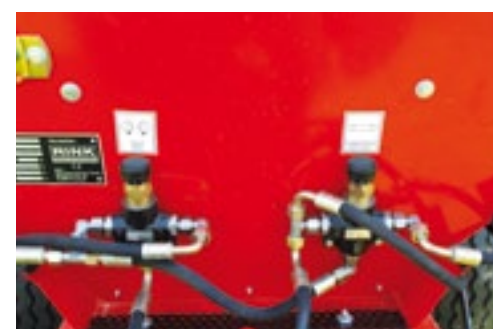
De Vibra Sandmaster drainmachine bestaat uit een schudfrees met een trillende zandbak om de sleuven te vullen met zand. Dit kan tot 17 cm diep. Zowel de frees als de trillende bak voor 1 kuub zand wordt mechanisch aangedreven. De rest, zoals heffen en de schuif van de bak opentrekken, gaat hydraulisch. Op het droge proefveld werden de sleuven goed tot 15 cm diep met zand gevuld. Wel ontstonden er opstaande randen naast de sleuven die je dan vlak moet rollen. Overigens waren er later bij een betere afstelling haast geen oneffenheden. Achterop zit een hele rij wielen om het gewicht van de machine te dragen. De Sandmaster kan 12 tot 15 kuub zand per 1.000 m 2 zand in sleuven brengen. Hij werkt 150 cm breed met sleuven op 26 cm afstand en kost 48.980 euro.
