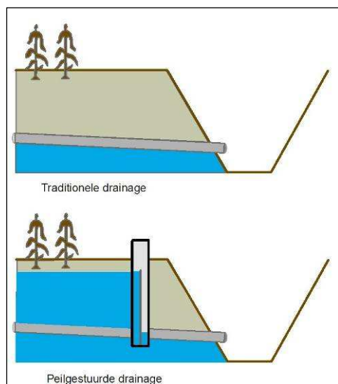
Figuur 4: Effect van peilgestuurde drainage op de grondwaterstand.
