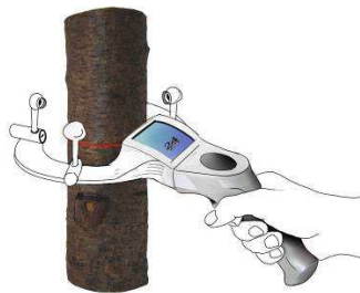
Laser driehoeksmeting
