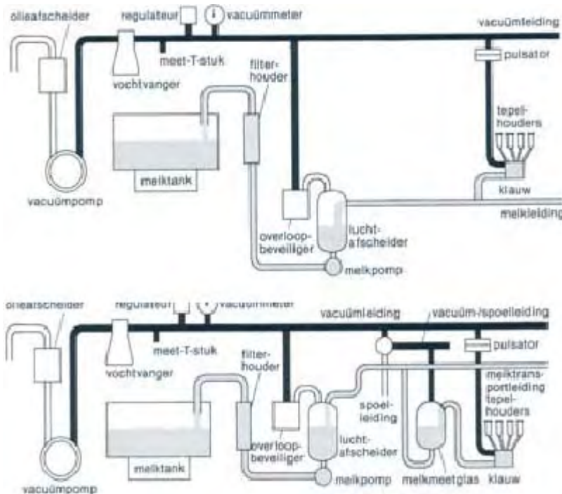
Figuur 9.1 Schematisch overzicht van een melkinstallatie met laagliggende melkleiding en van een melkinstallatie met melkmeetglazen (onder)
