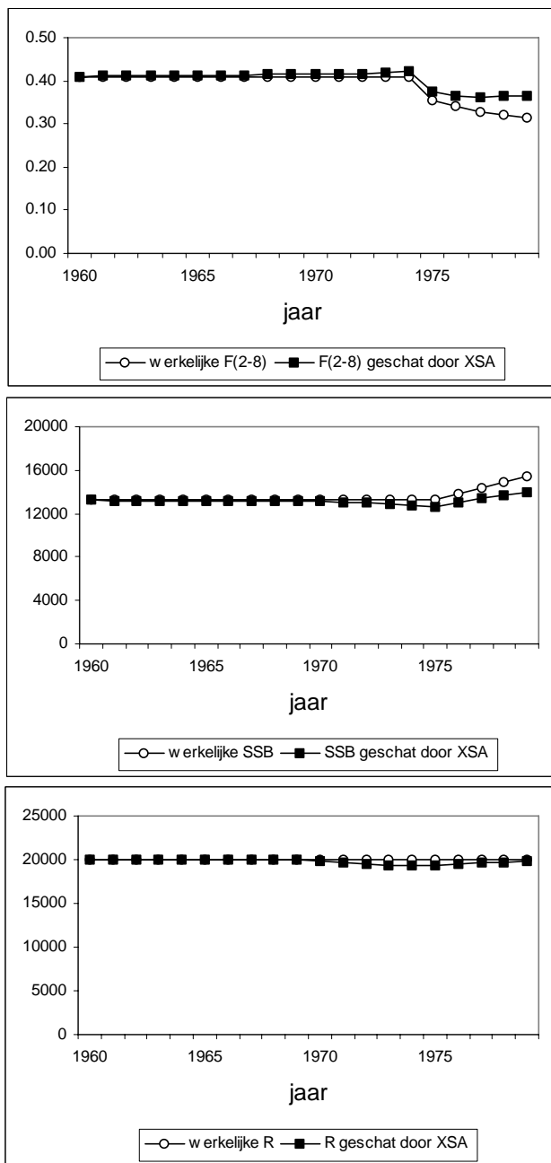
Figuur 6. Simulatiemodel 2 met een kalibratieserie waarvan de survey slechts deelgebied 1 beslaat. De werkelijke en de door XSA geschatte toestand van het bestand. Boven F_{2,8} . Midden SSB (eenheden niet van belang). Onder R in aantallen.
