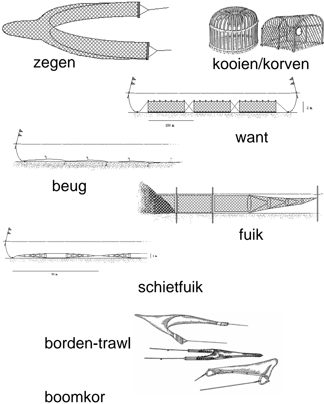
Figuur 1. Overzicht van vangstuigen die worden gebruikt in de kleinschalige Nederlandse kustvisserij.
