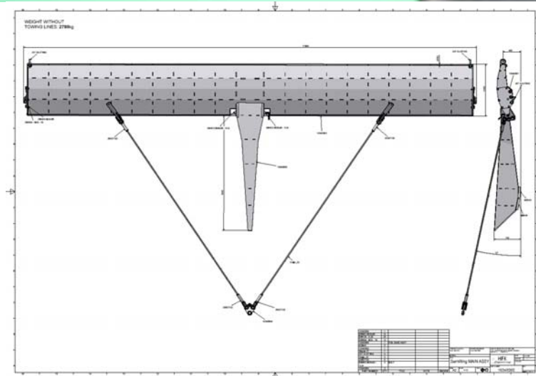
Figuur 16. Zweefkor - "Sumwing" constructie; Foto: Sumwing, zonder zijanten, met foam.
