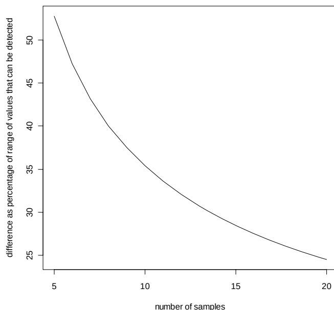
Figuur 1. Resultaat poweranalyse zandsuppletiegegevens (data Van der Wal & Van Dalfsen 2008): x-as: aantal monsters per gebied. Y-as: te detecteren verschil tussen gebieden met significantie 0.05 en power van 0.8 (log-getransformeerde gegevens).
