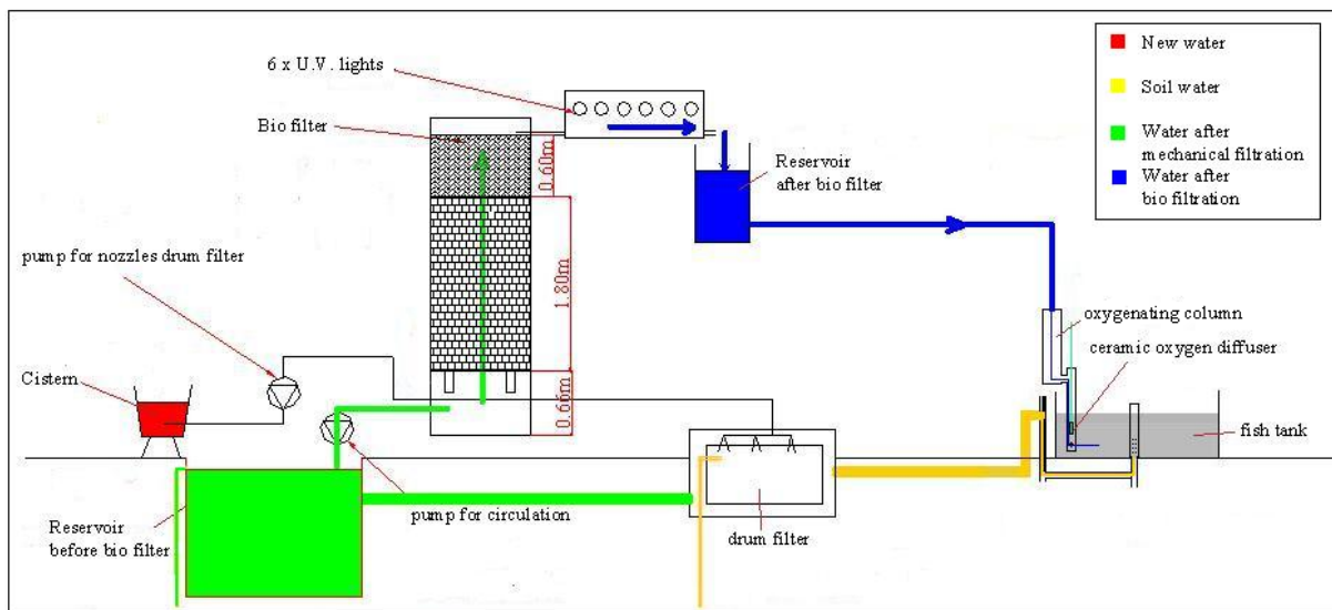
Fig. 6.3 Schematische weergave van het recirculatiesysteem.
