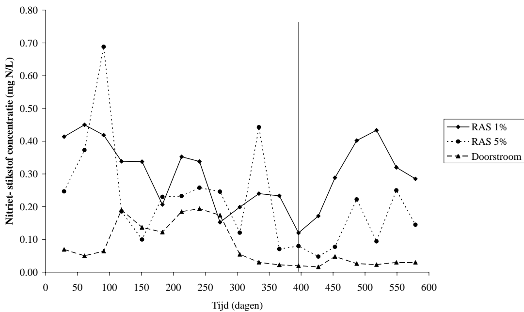
Fig. 6.14. Maandelijks gemiddelde van de nitriet-stikstofconcentratie in het water van de drie kweeksystemen. De verticale lijn geeft het tijdstip aan waarop de systeemverversing van RAS1% verlaagd is.
