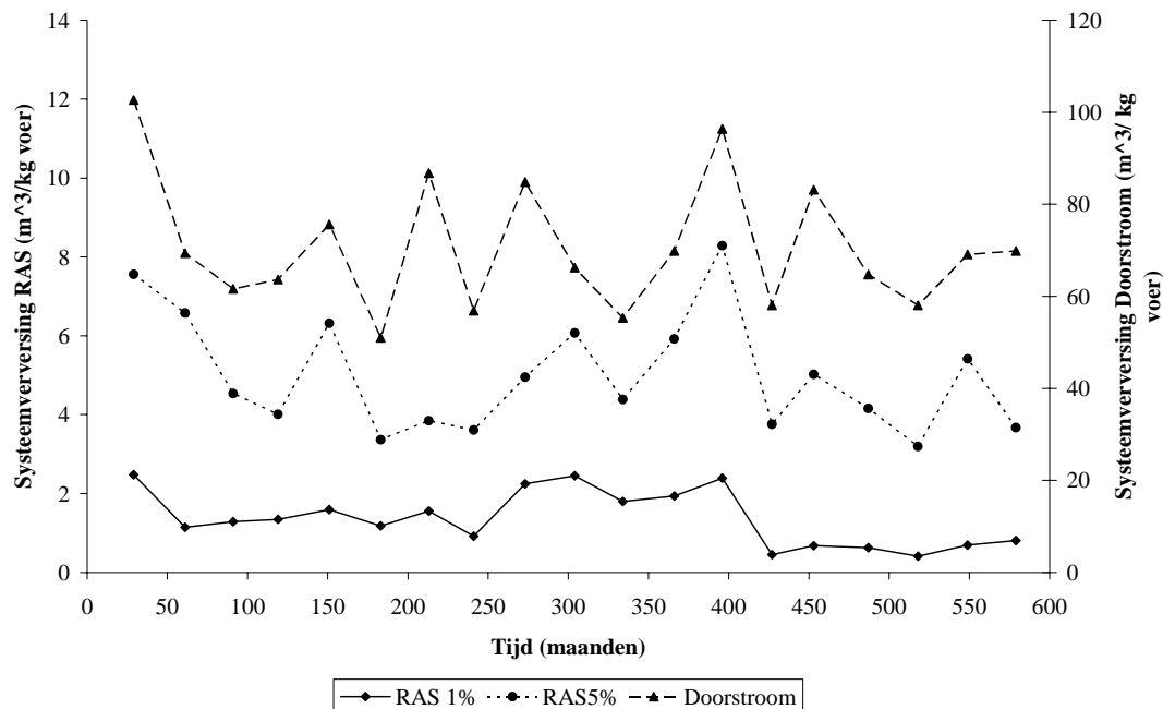
Fig. 6.1 De mate van verversing van de experimentele kweeksystemen gedurende het experiment uitgedrukt in (m 3 /kg voer). De linker X-as betreft de twee recirculatiesystemen. De rechter X-as betreft het doorstroomsysteem.
