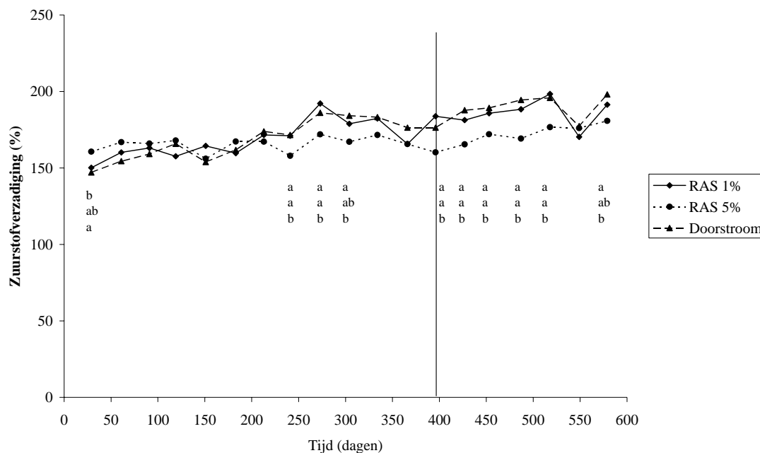
Fig. 6.10 Maandelijks gemiddelde zuurstofverzadiging (n = 20) in het water van de drie kweeksystemen. Meetwaarden gemarkeerd met verschillende letters verschillen significant (P < 0.05). De verticale lijn geeft het tijdstip aan waarop de systeemverversing van RAS1% verlaagd is.
