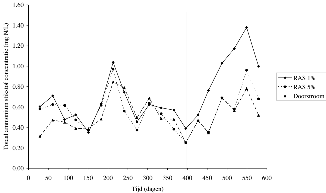
Fig. 6.13. Maandelijks gemiddelde van de concentratie totaal ammonium stikstof (TAN) in het water van de drie kweeksystemen. De verticale lijn geeft het tijdstip aan waarop de systeemverversing van RAS1% verlaagd is.
