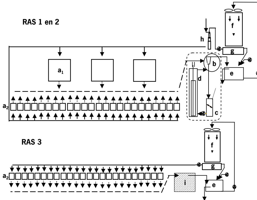
Figuur 2.1. Schema van RAS 1, 2 en 3 zoals gebruikt in dit experiment. In RAS 1 en 2 stroomt water als volgt: de kweektanks (a 1 ) /experimentele tanks (a 2 ) – drum filter (b) – buffer tank (c) – denitrificatie reactor (d) – drum filter (b) – reservoir 1 (e) – trickling filter (f) – reservoir 2 (g) – zuurstofreactor (h) – kweektanks/experimentele tanks (a 1 ). In RAS 3 stroomt water als volgt: experimentele tanks (a 1 ) – plaatbezinker (i) – reservoir 1 (e) – trickling filter (f) – reservoir 2 (g) – experimentele tanks (a 1 ).
