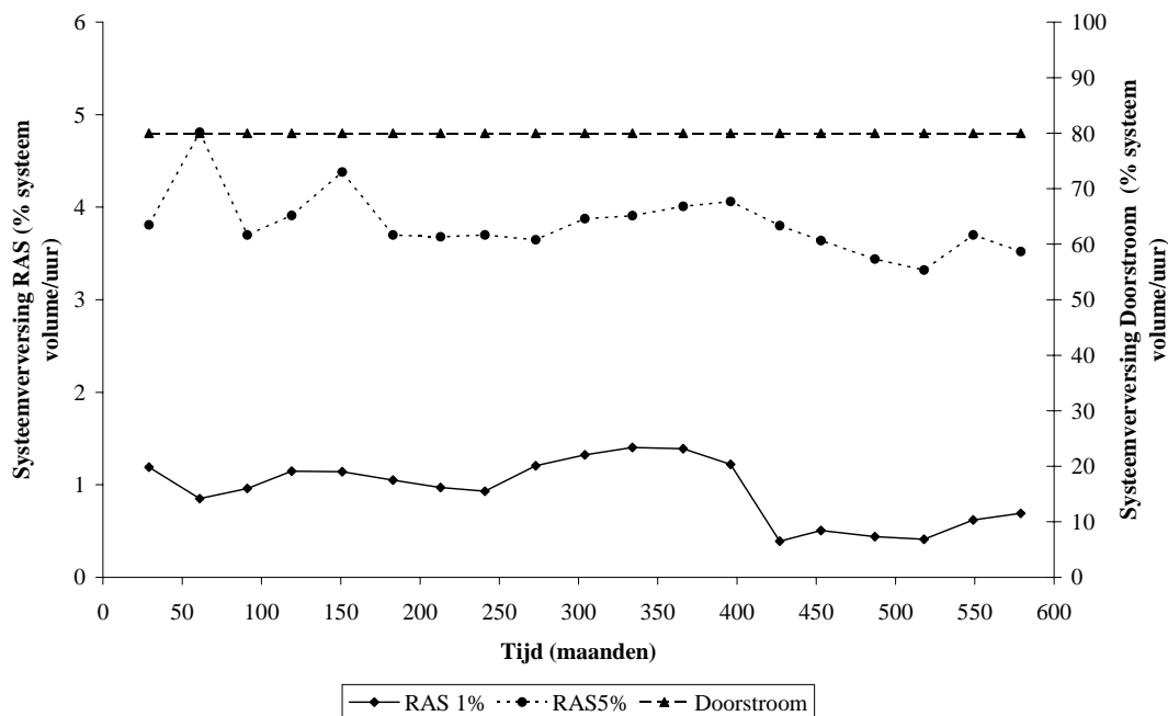
Fig. 6.2 De mate van verversing van de experimentele kweeksystemen gedurende het experiment uitgedrukt in (% systeemvolume/uur). De linker X-as betreft de twee recirculatiesystemen. De rechter X-as betreft het doorstroomsysteem.
