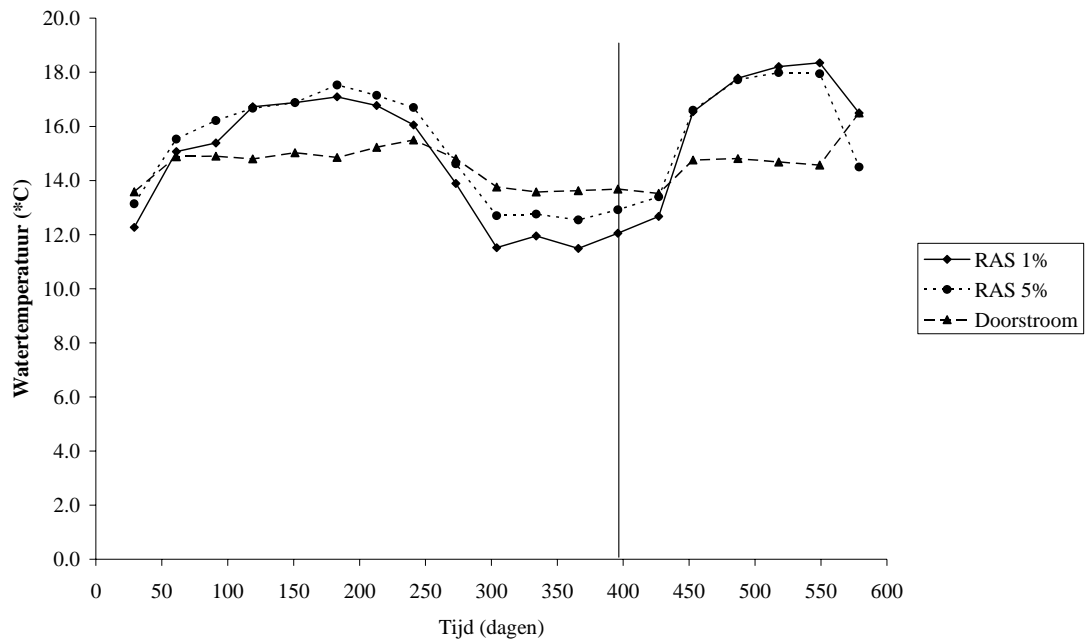
Fig. 6.11 Maandelijkse gemiddelde watertemperatuur (n = 20) van de drie kweeksystemen. De verticale lijn geeft het tijdstip aan waarop de systeemverversing van RAS1% verlaagd is.
