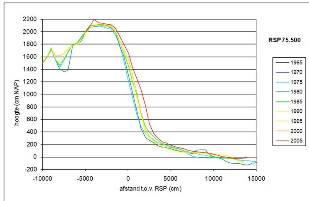
Figuur 6.12. Typerend dwarsprofiel voor Langeveld.
