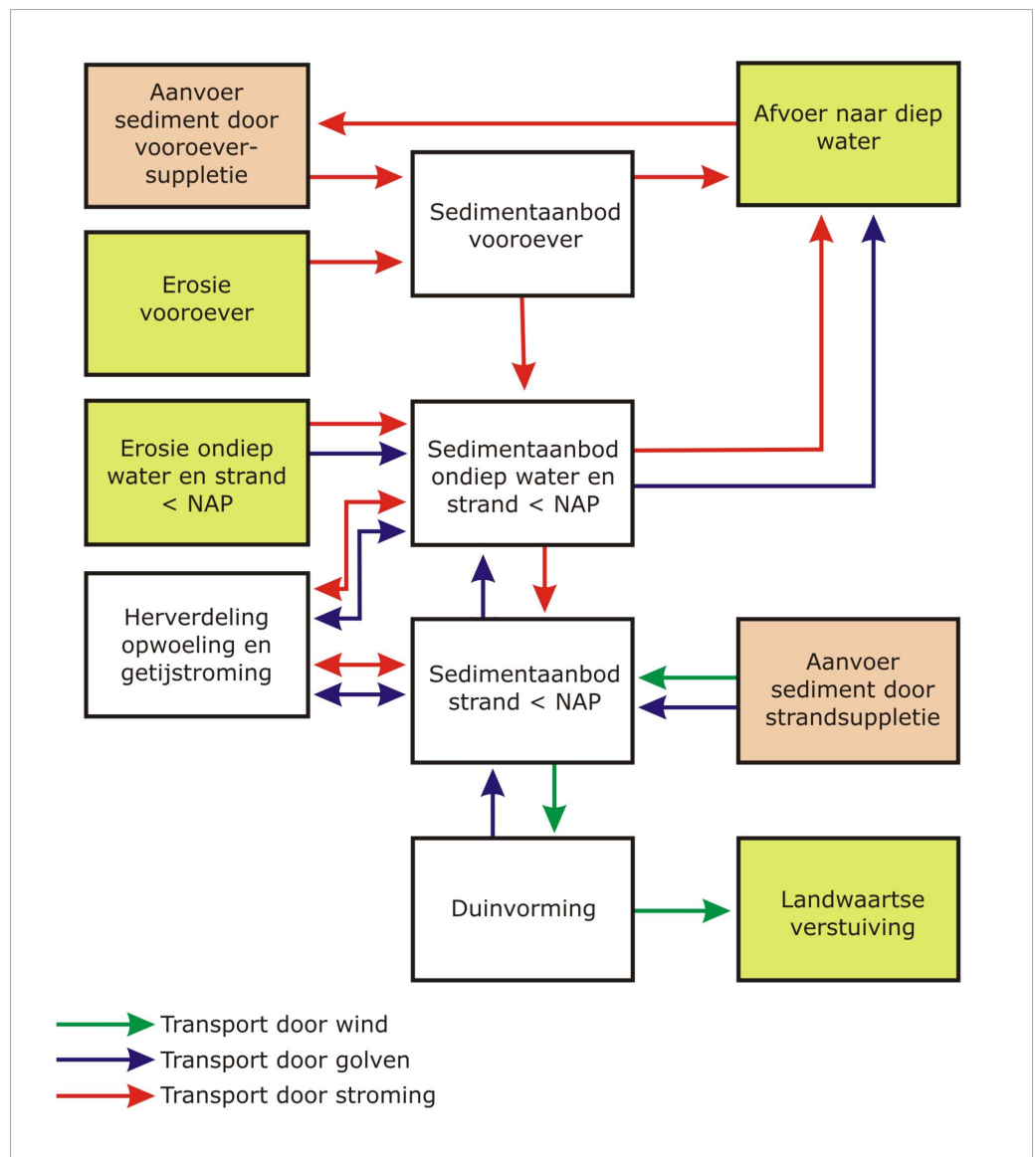
Figuur 2.1. Effecten van suppleties op processen op vooroevers, strand en duinen. Naar Jeuken et al, 2005.
