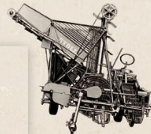
Stoll B.R.S. 2-B20 bietenrooier met bunker.
