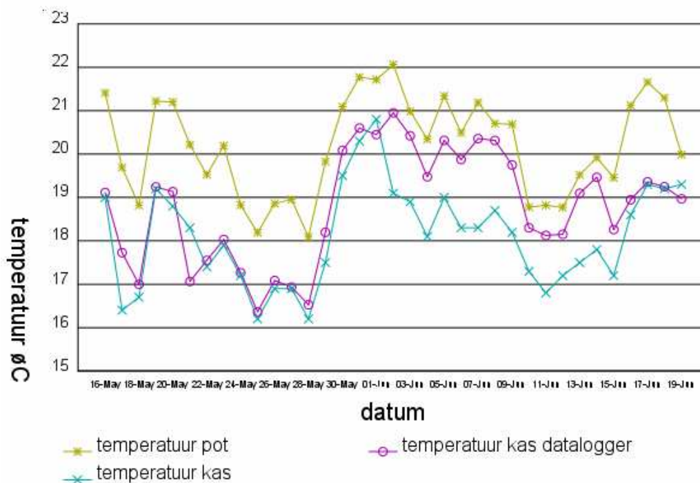
Figuur 18 Het temperatuurverloop in de tijd in kasproef 1990 in de lucht en in de potten
