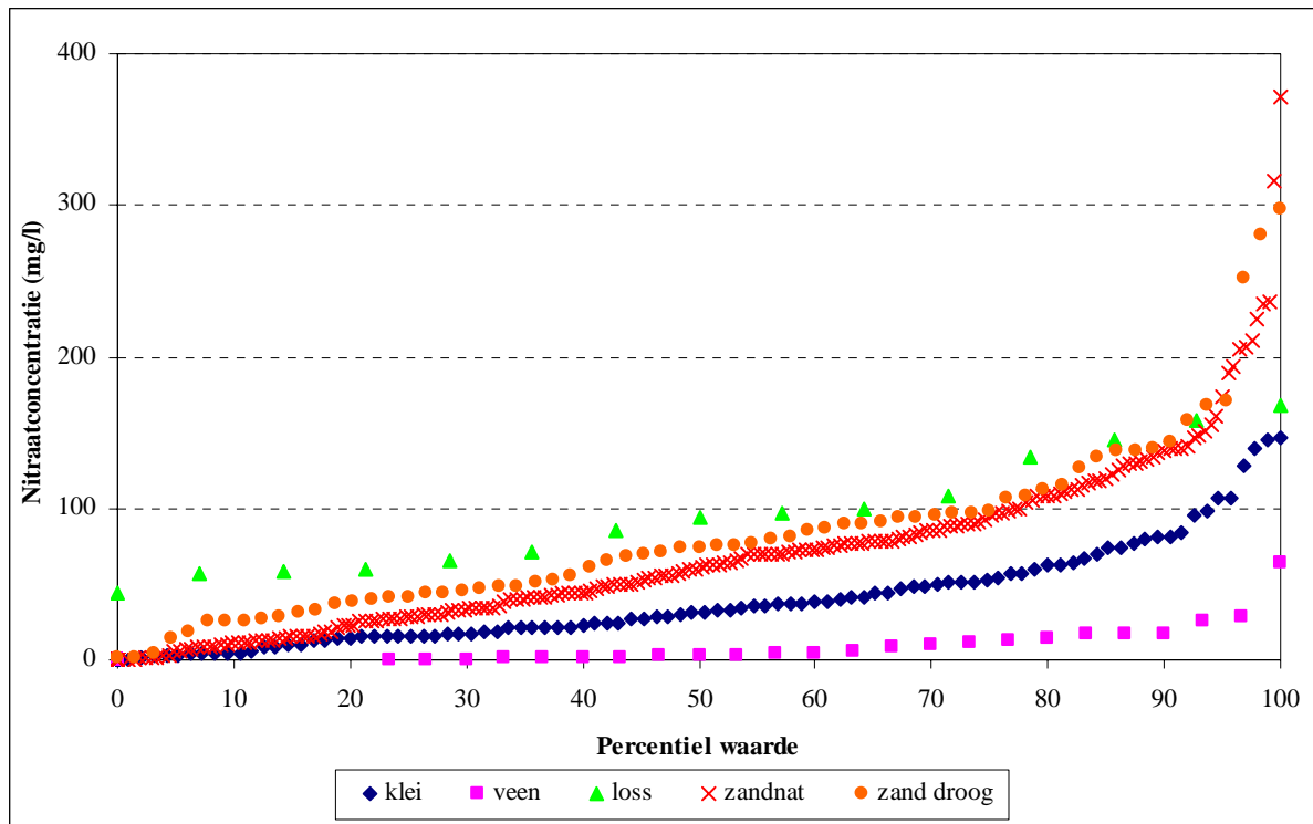
Figuur 2: Percentielgrafiek voor de nitraatconcentratie in de verschillende hoofdgrondoorstroomregio's (gemiddelde 2002-2004)
