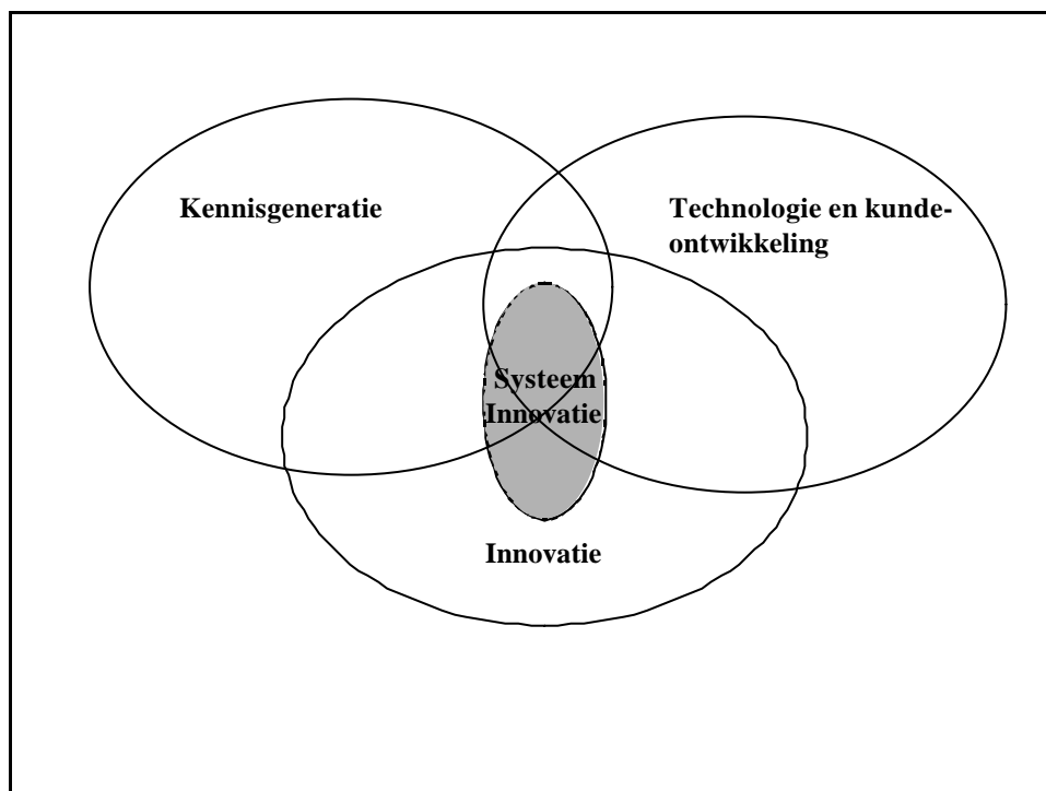
Figuur 4: LAT-model
