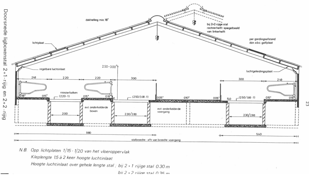
Figuur 1: Dwarsdoorsnede van een veel gebouwd type ligboxenstal zoals beschreven in de RICHTLIJNEN VOOR DE BOUW EN INRICHTING VAN LIGBOXENSTALLEN (Bron: 1988, Consulentenschap in Algemene Dienst voor de Bedrijfsuitrusting in de Veehouderij).
