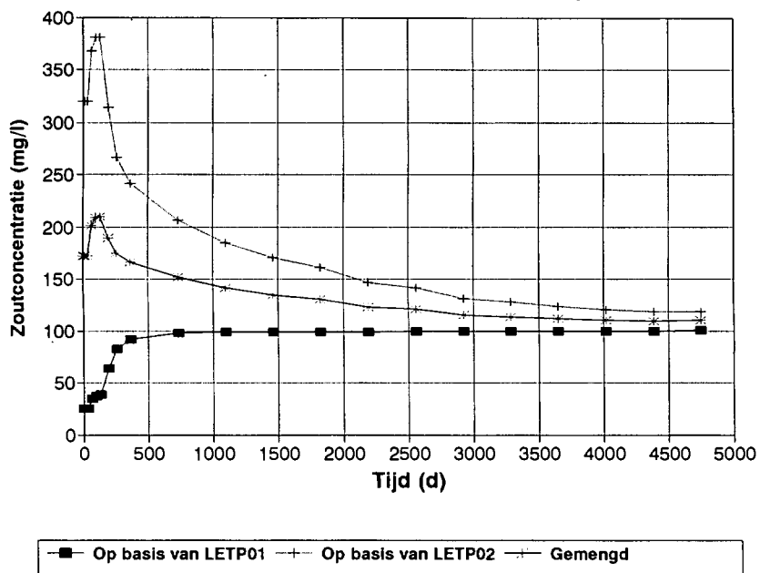
Figuur 5: Berekend zoutconcentratie-verloop
