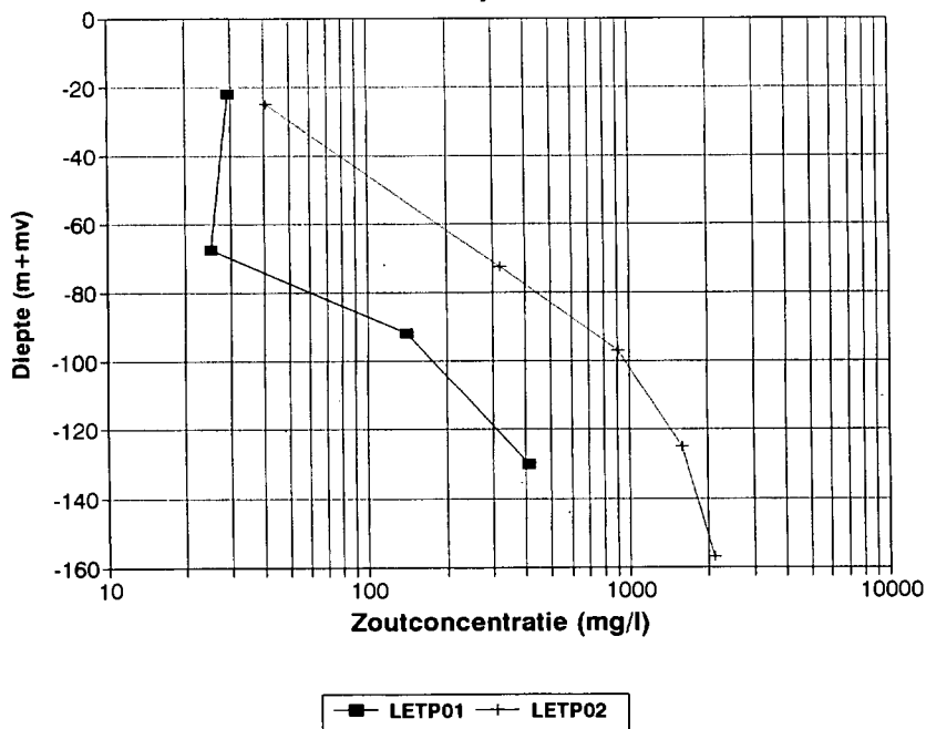
Figuur 4: Gemeten zoutconcentratie profielen Lettele
