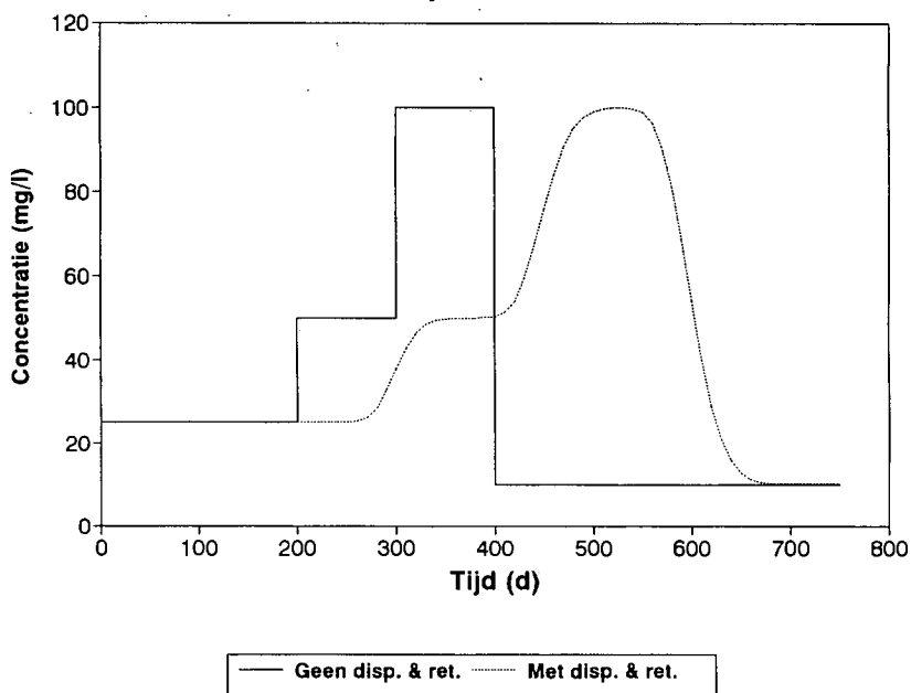
Figuur 3: Effect van dispersie en retardatie op het concentratieverloop van het opgepompte grondwater
